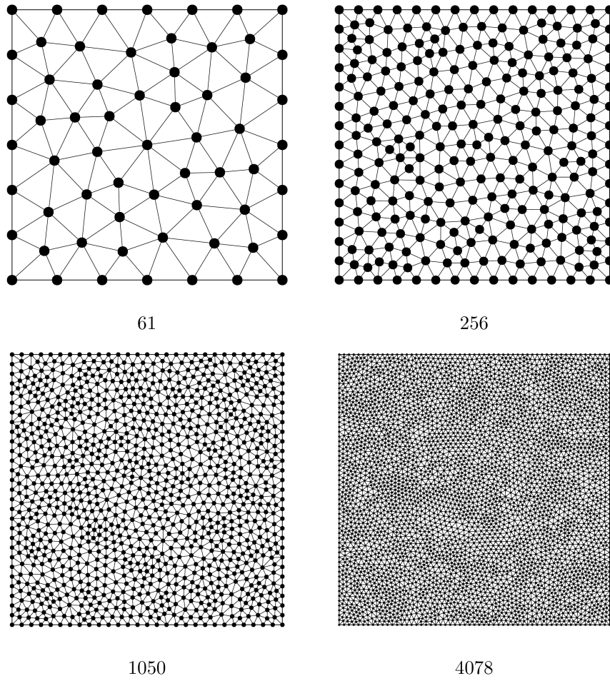
图 4.2 固支方板挠度场的节点布置（图中数字为节点数）
