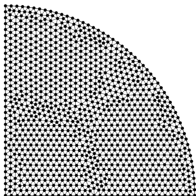
图 4.7 固支圆板问题节点离散
