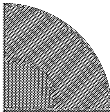
图 4.7 固支圆板问题节点离散
