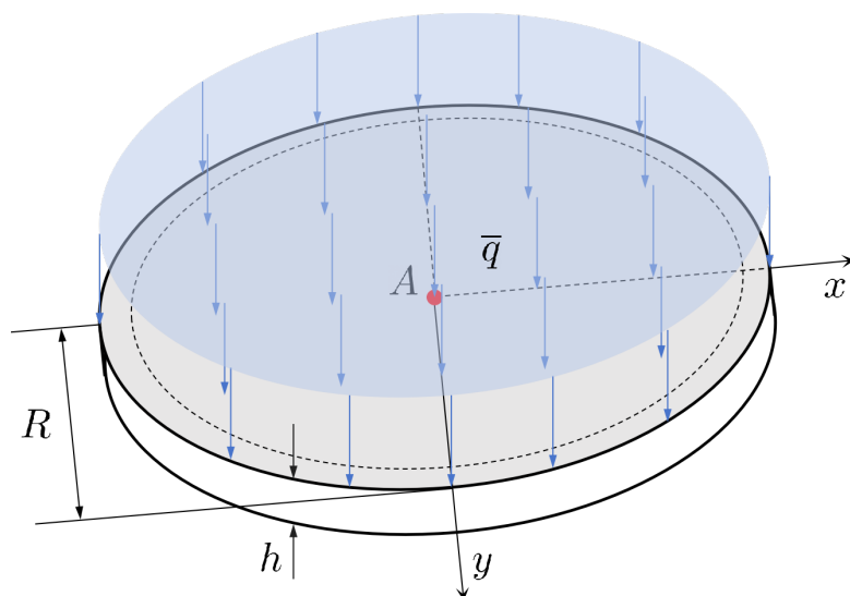
图 4.6 周边固支圆板示意图
