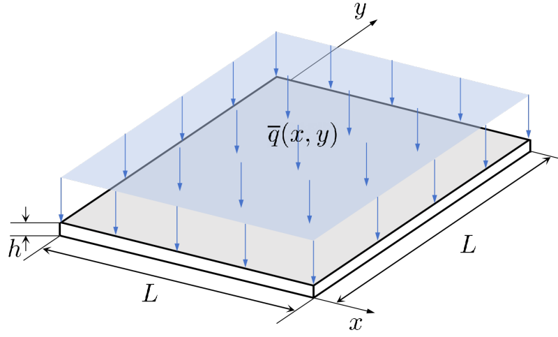
图 4.1 四边固支方板示意图
