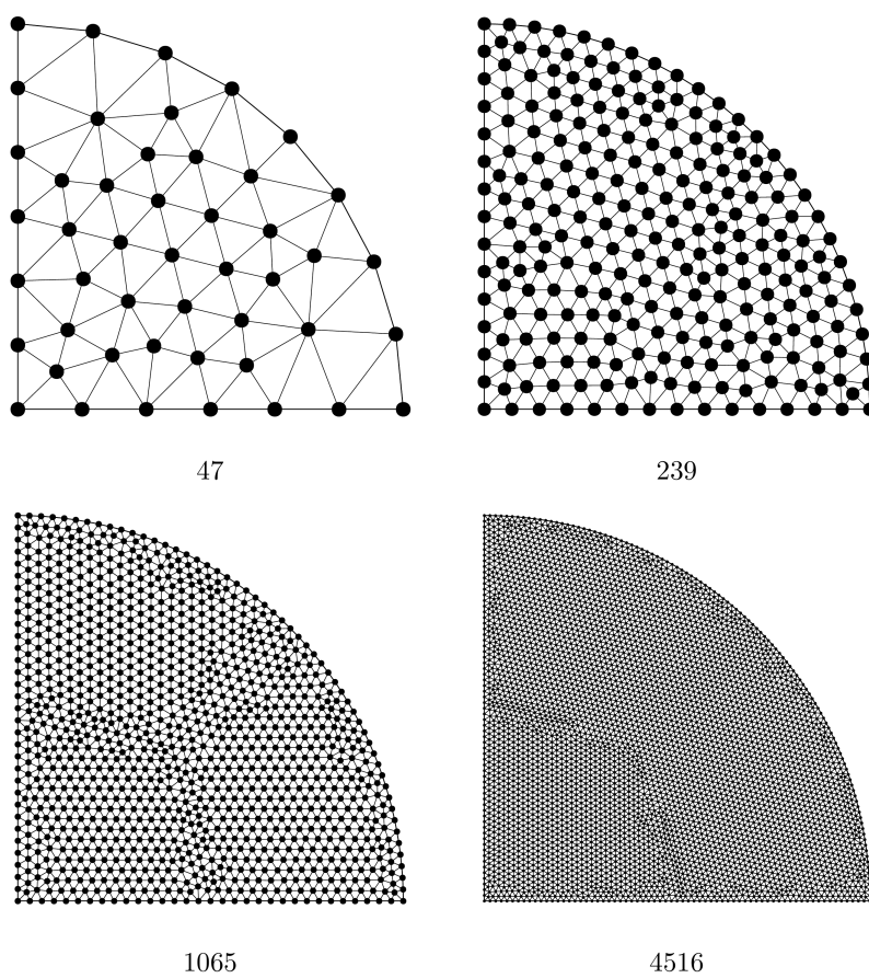
图 4.7 固支圆板挠度场的节点布置（图中数字为节点数）
