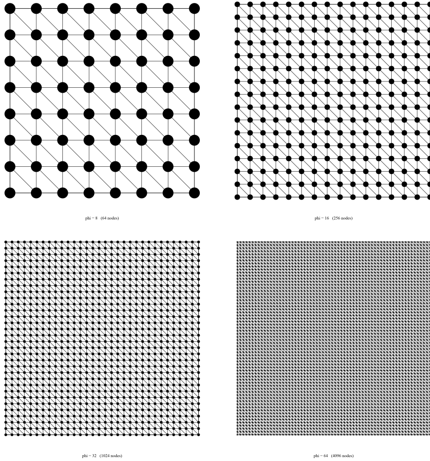
图 4.2 固支方板挠度场的节点布置（图中数字为节点数）
