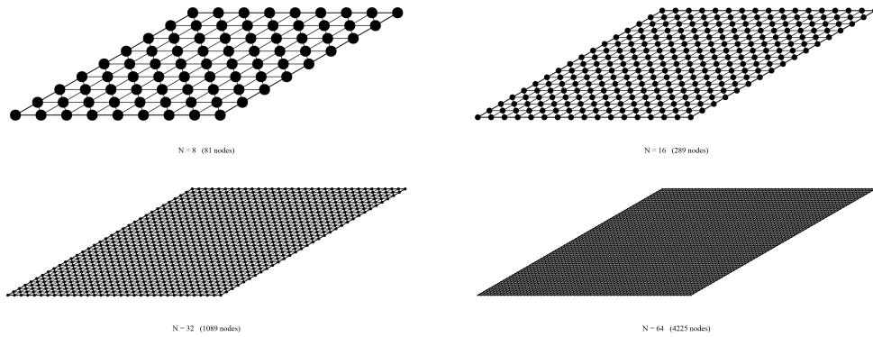
图 4.9 锐角斜板挠度场的节点布置（图中数字为节点数）
