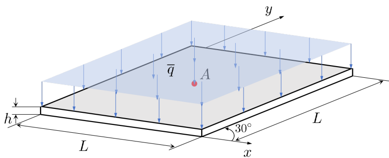
图 4.8 菱形锐角斜板示意图
