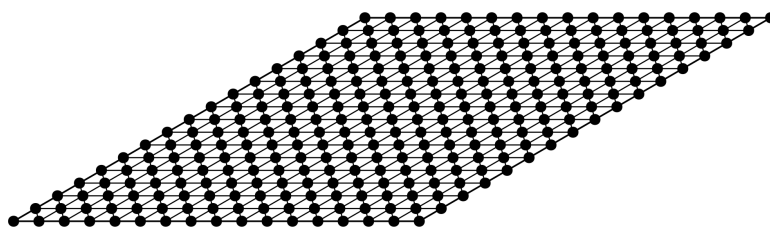
图 4.9 斜板问题节点离散
