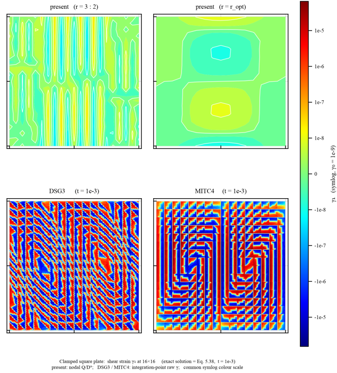
图 4.3 固支方板剪切应变 \gamma_1 的等值线云图（ 16 \times 16 网格，统一色标）
