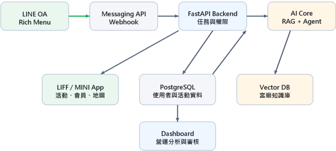
圖1：Temple AI OS 系統架構圖
