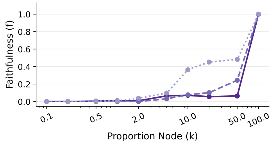
Llama-3
