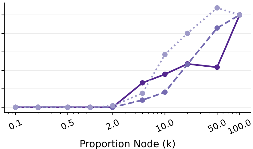
Qwen-2.5
