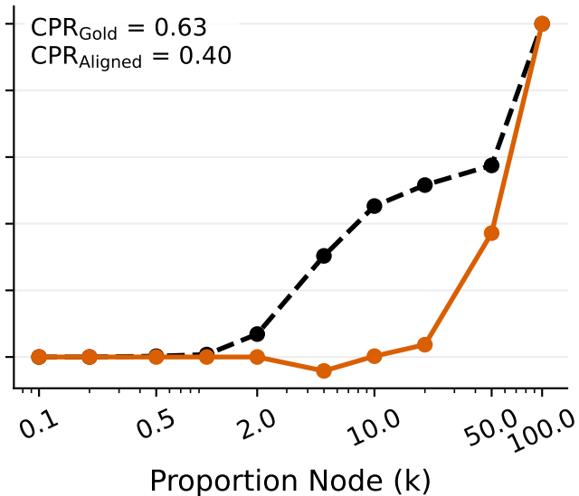
Llama-3 1B \rightarrow 8B
