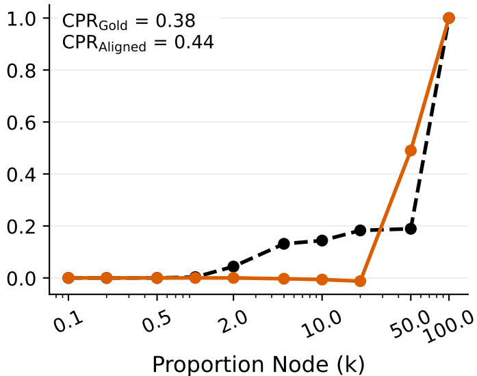
Llama-3 1B \rightarrow 3B
