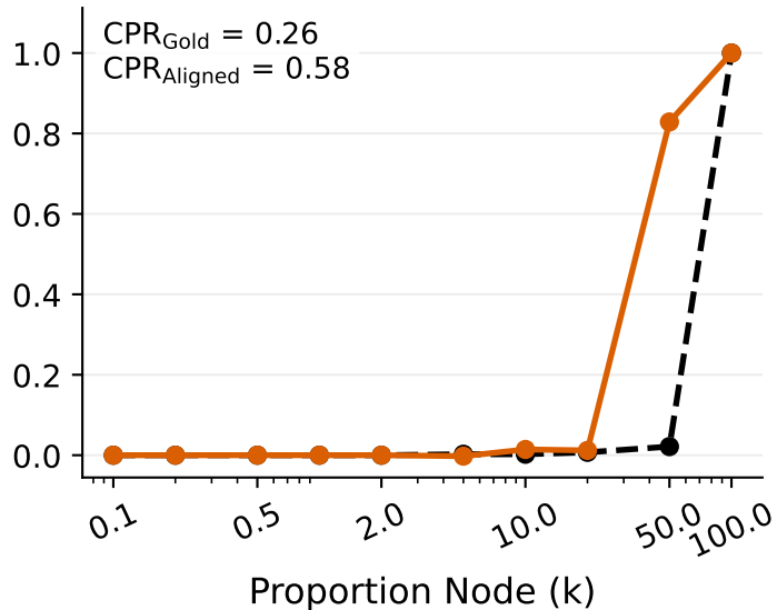
Llama-3 1B → 3B
