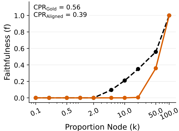
Qwen-2.5 0.5B → 1.5B
