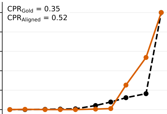
MCQA
