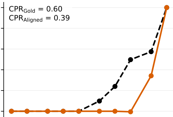
MCQA
