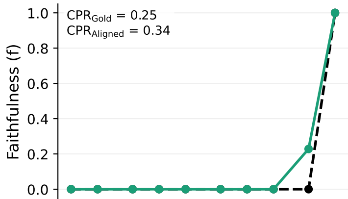
IOI
