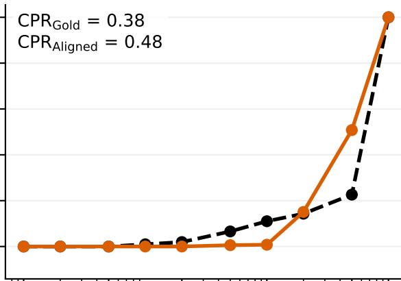
MCQA
