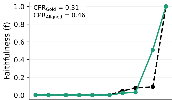
IOI
