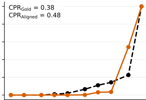
MCQA
