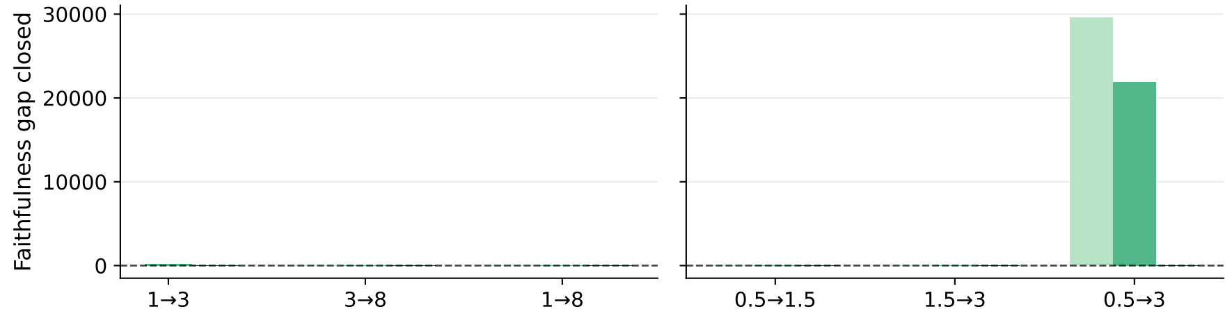
Qwen-2.5
