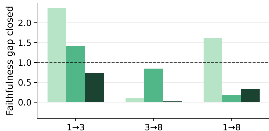
Llama-3
