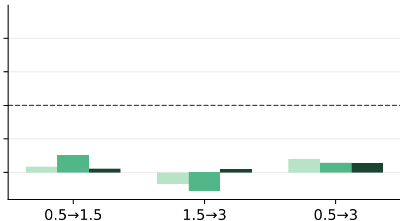
Qwen-2.5
