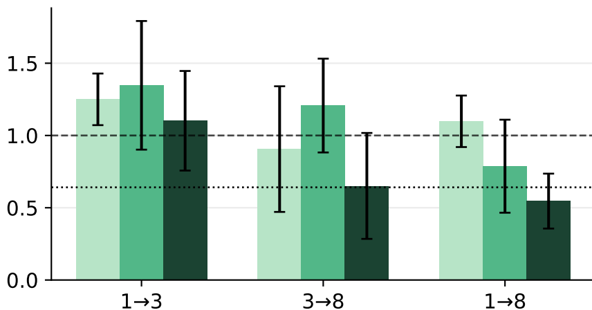
Llama-3
