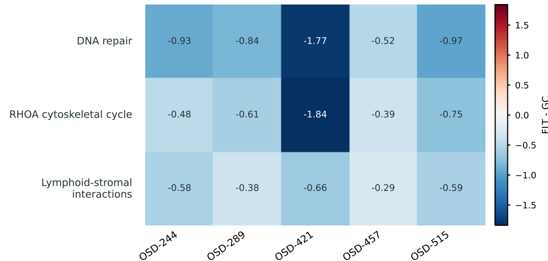
A Thymus
