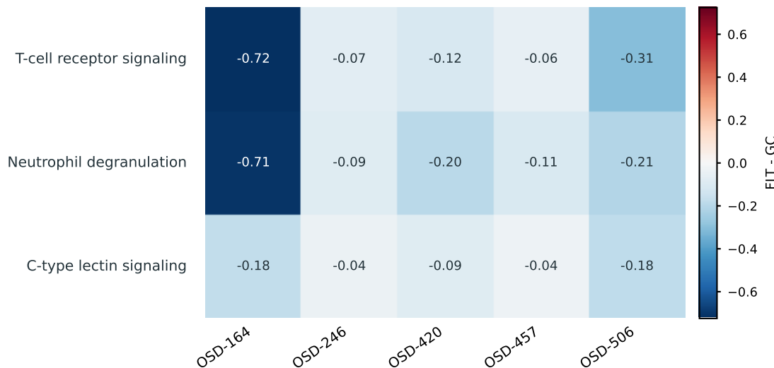
C Spleen
