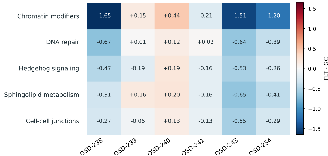
B Skin
