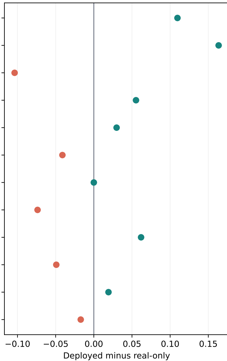
AUROC
