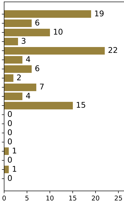
Notagen (n=100)
