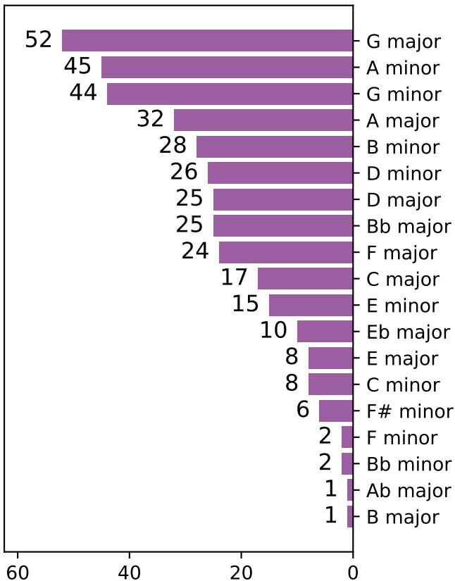
Bach (n=371)
