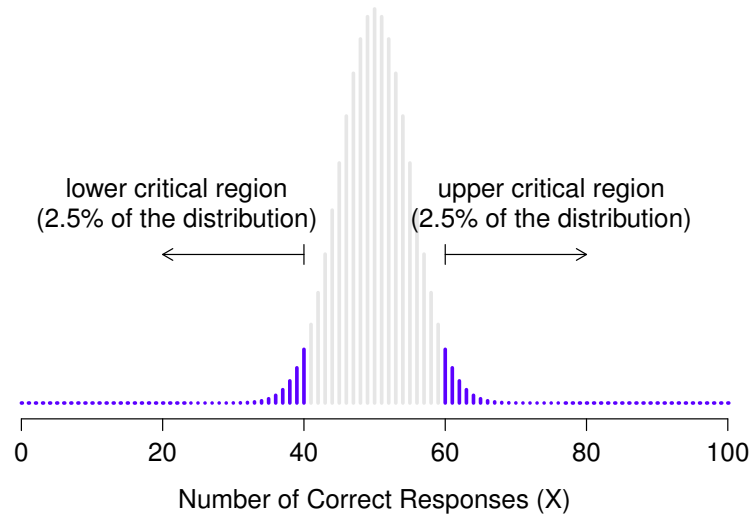
Figure1.2 有意水準 \alpha = .05 の検定における，ESP 研究の仮説検定の棄却域。図は帰無仮説のもとでの X の標本分布（つまり図 ?? と同じもの）を示している。灰色のバーは帰無仮説を保持することになる X の値，青い（濃い）バーは帰無仮説を棄却することになる X の値，すなわち棄却域である。対立仮説は両側（ \theta < .5 と \theta > .5 の両方を許す）なので，棄却域は分布の両裾を覆う。 \alpha 水準を .05 にするには，2 つの領域がそれぞれ標本分布の 2.5% を含むようにする必要がある。
