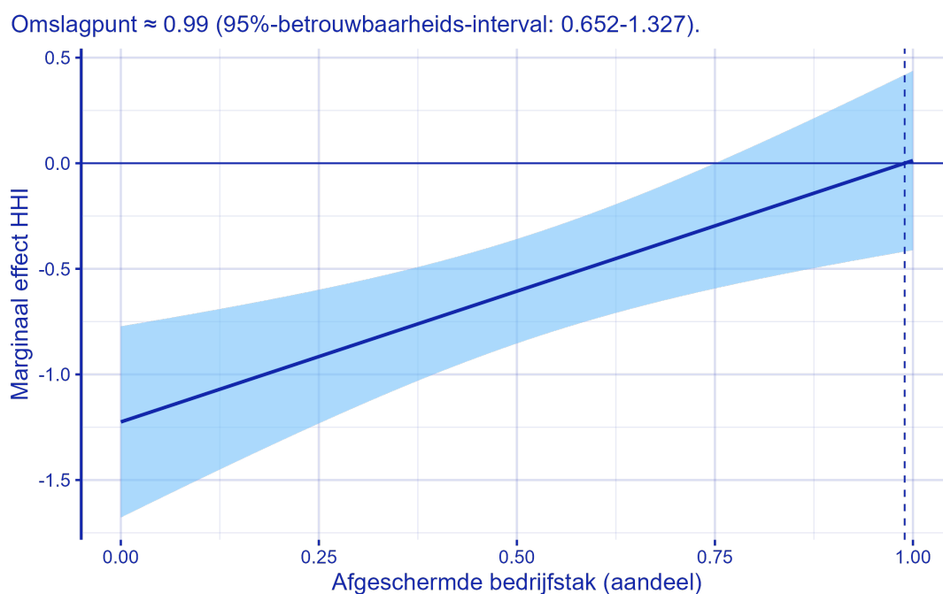
Figuur 1: Interactie-effect Marktconcentratie (HHI) \times Afgeschermded bedrijfsta (aandeel)
