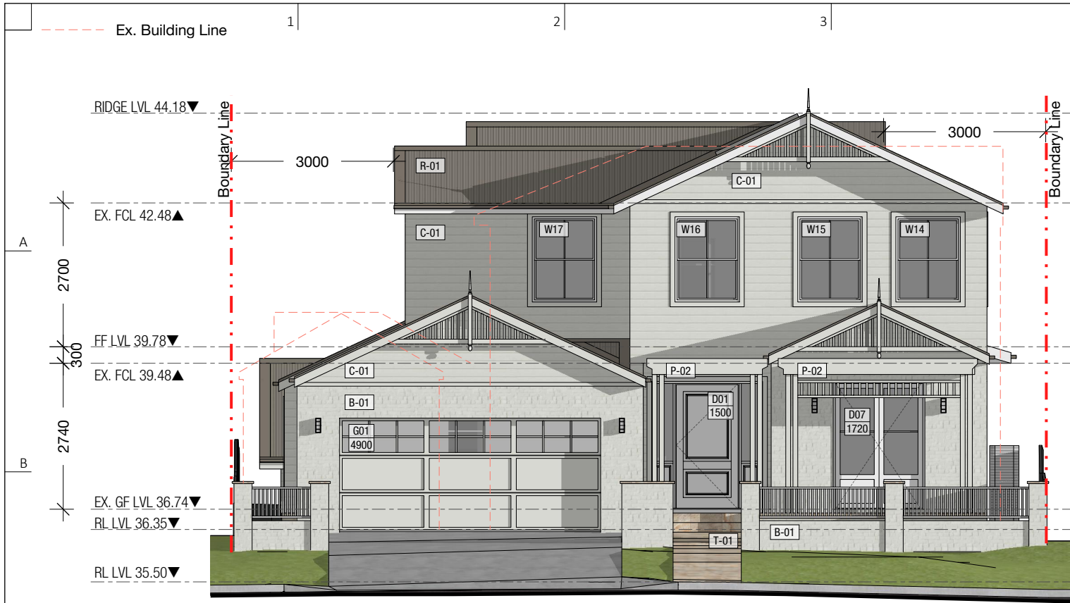
C1 South Elevation SCALE: 1:100
