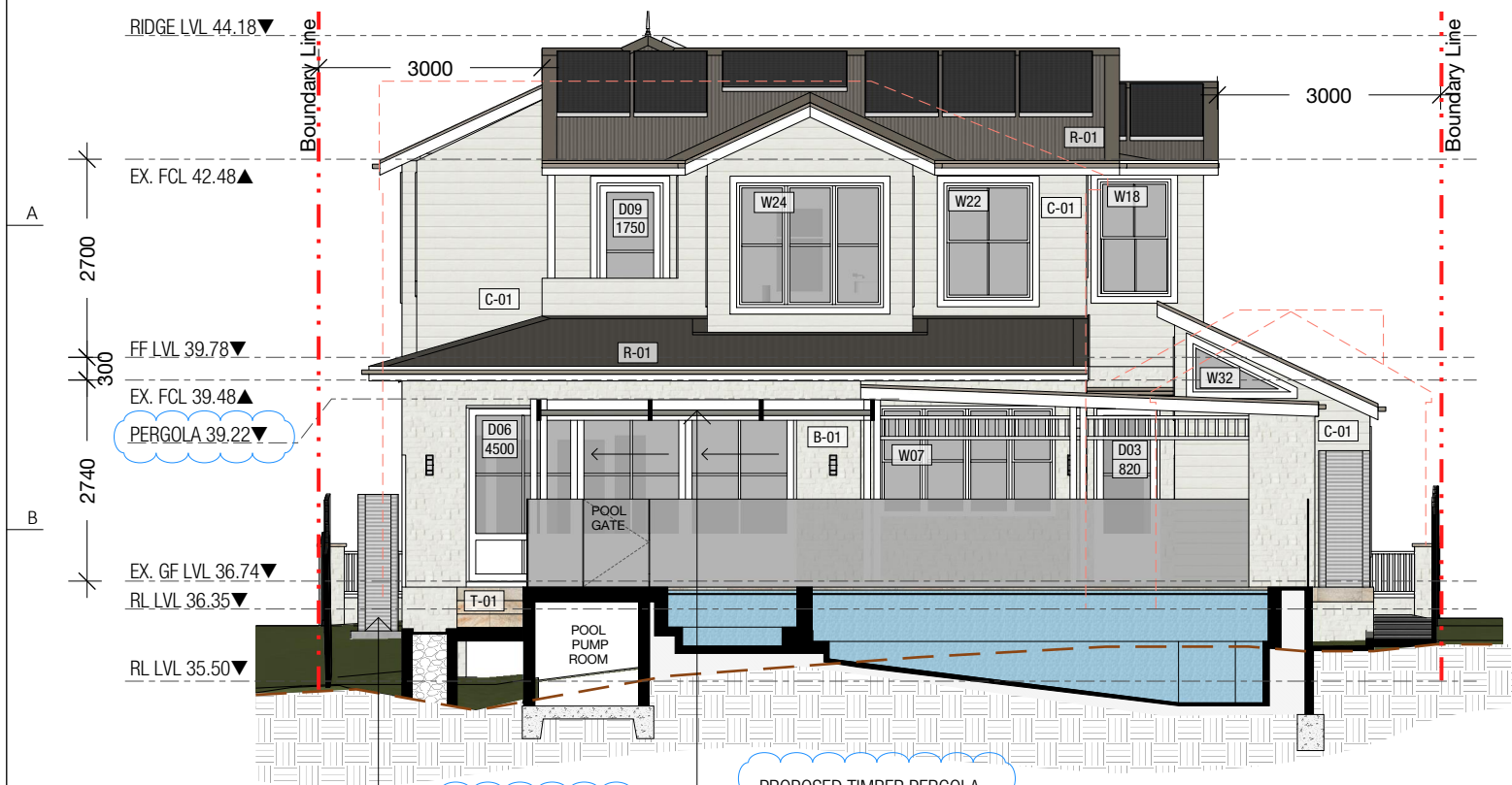
C1 North Elevation SCALE: 1:100
