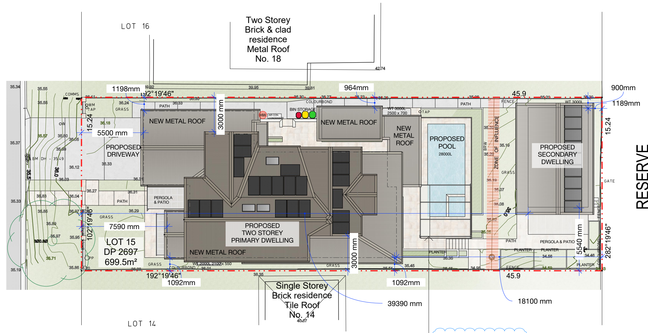
C1 Site Plan SCALE: 1:200
