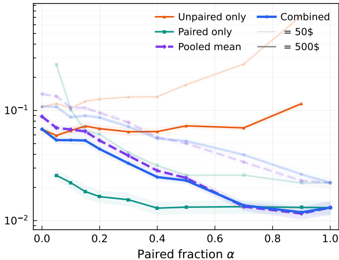
Off-diagonal MSE
