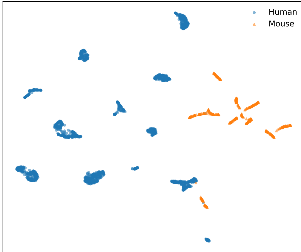
ESPRESSO: species
