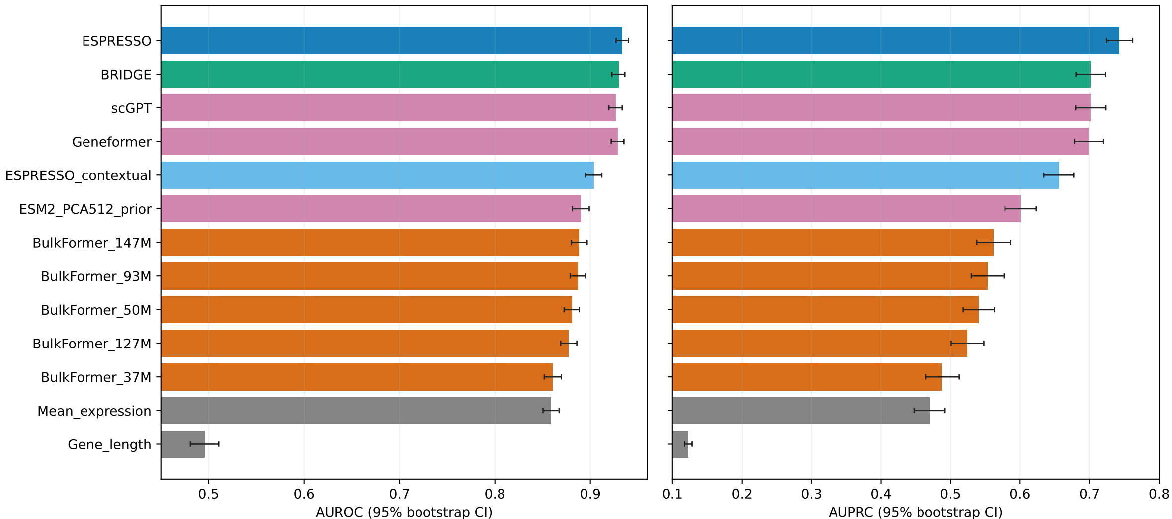
AUROC
