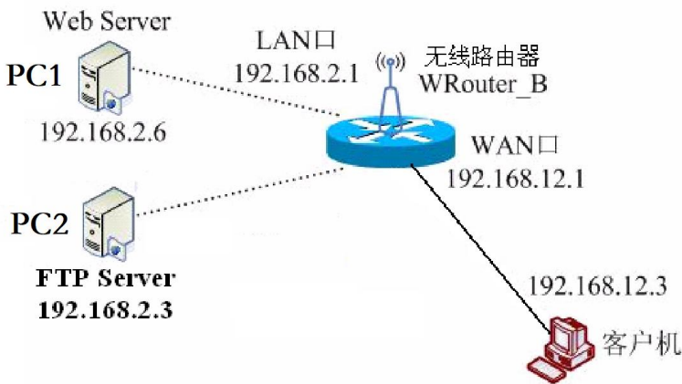
网络拓扑图
