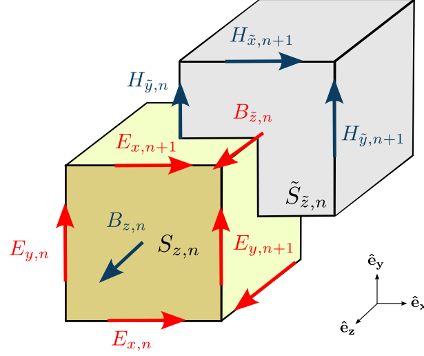
Fig. 3.3: Celda V_n del complejo G y celda dual \tilde{V}_n del complejo \tilde{G} desplazada media celda en todas las direcciones y ortogonal a la primera. Se muestran las cantidades asociadas a una cara S_{z,n} y \tilde{S}_{\tilde{z},n} del complejo G y \tilde{G} , respectivamente. Se muestran en azul las cantidades relacionadas con los campos magnéticos y en rojo con los campos eléctricos.
