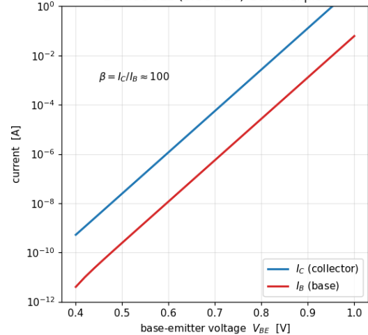
B. HICUML2 (SiGe HBT) Gummel plot
