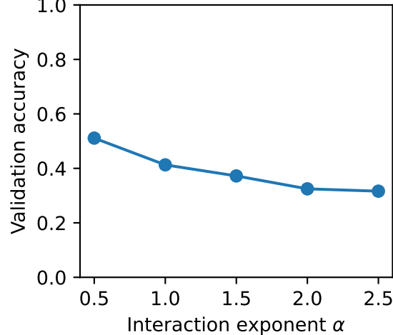
(d) Accuracy vs \alpha
