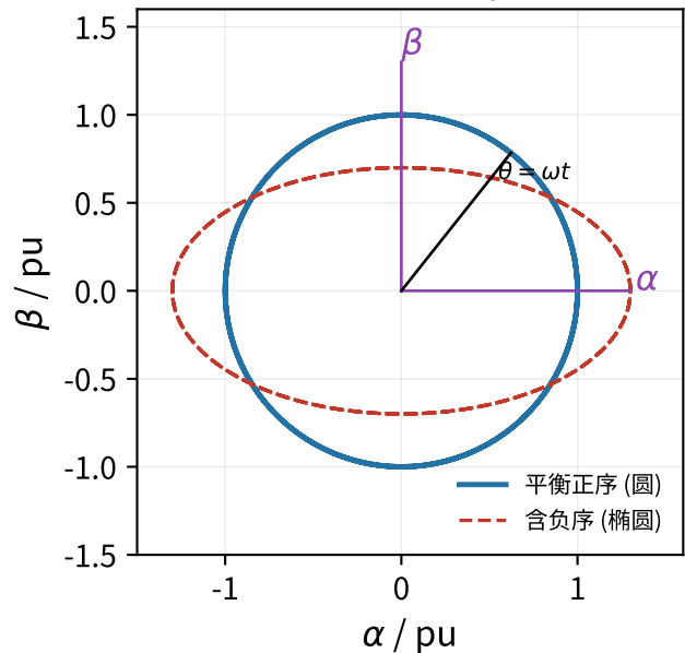
(c) \alpha\beta 轨迹: 旋转矢量在 dq 系中成为常矢量
