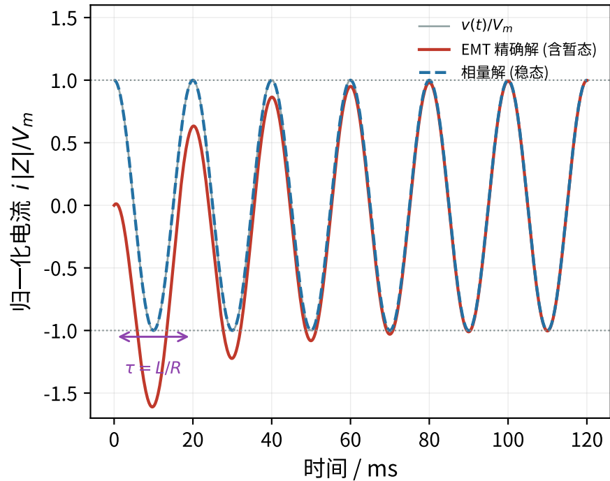
(a) 最坏合闸相角 \phi = \phi_z : 相量法缺失的暂态与稳态同量级
