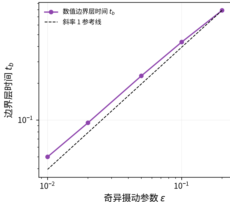
(c) 快动态时间 \propto \varepsilon : \varepsilon \rightarrow 0 即降阶
