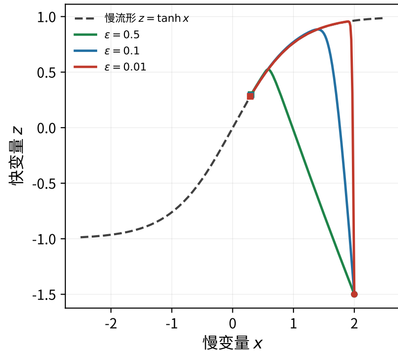
(a) 相平面: 先到慢流形, 再沿岸演化
