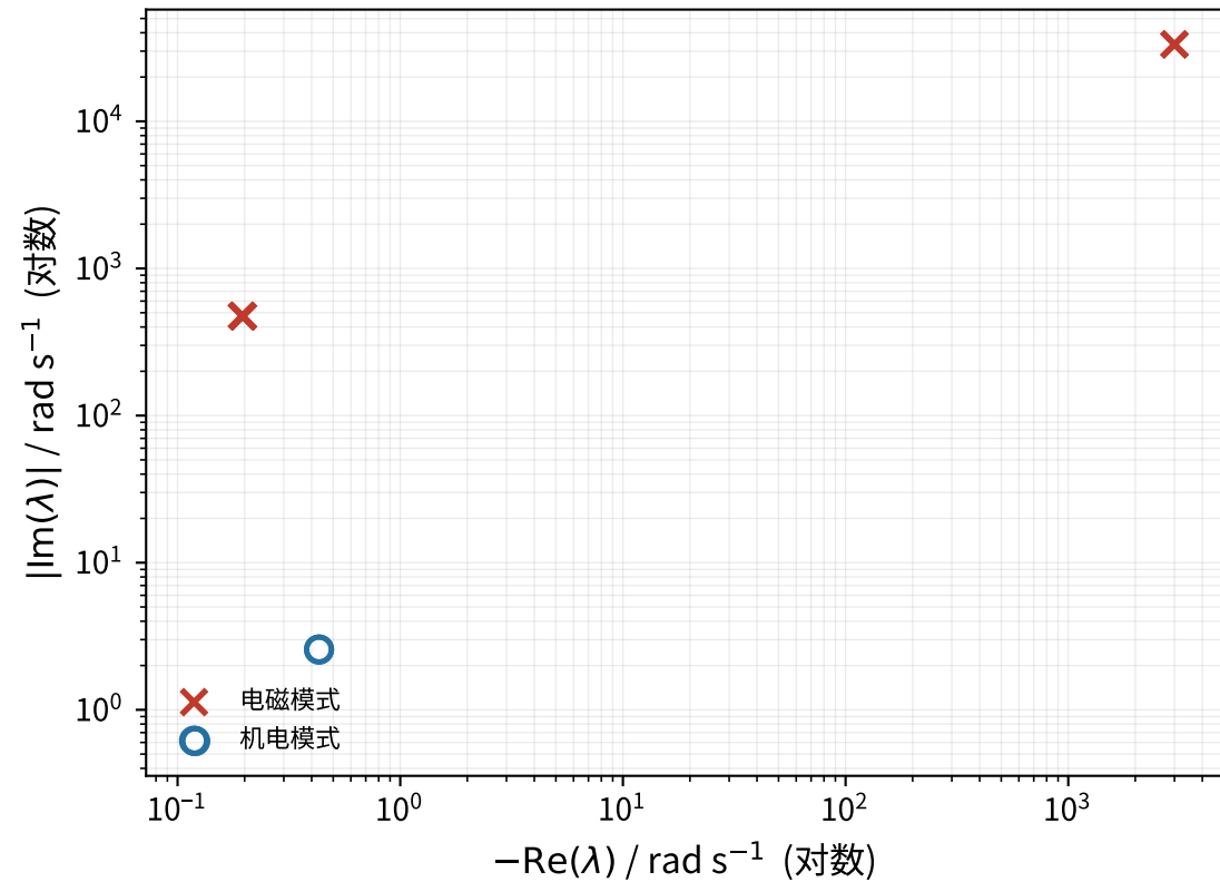
(a) 特征值分布 (双对数): 两团相距 4~5 个数量级
