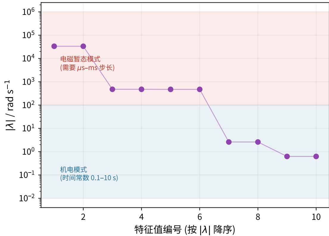
(b) 刚度比 \approx 5.4\text{e}+04 : 快慢模式相差 5 个数量级
