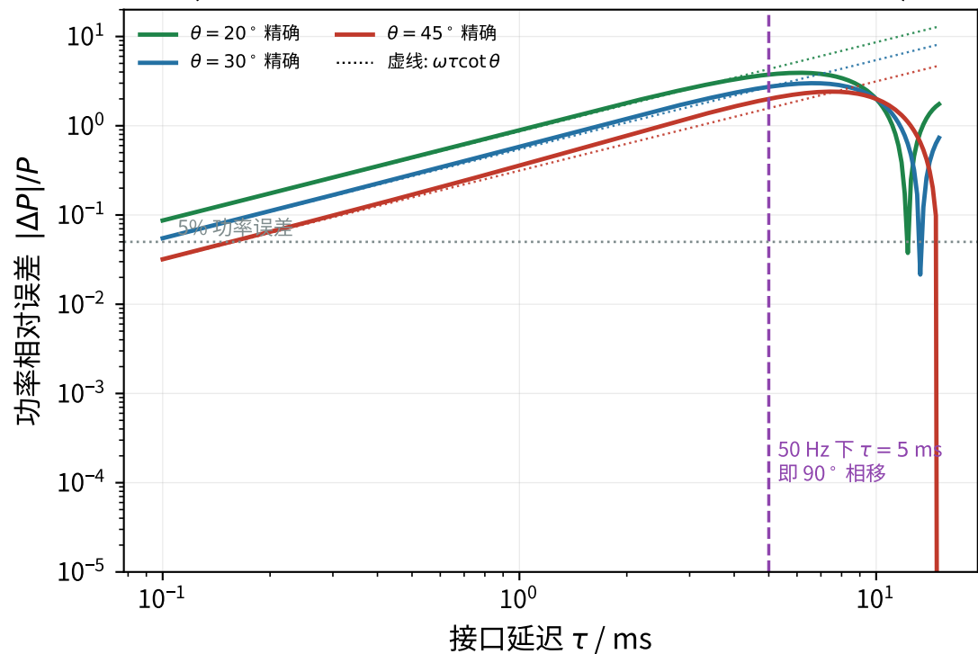
(b) 接口延迟导致的功率误差: 小延迟下 \approx \omega \tau \cot \theta (注: \tau = 20 \text{ ms} 的整周期延迟对单一频率反而无误差)
