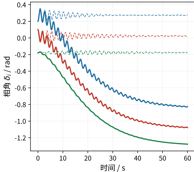
(b) R/X = 0.5 : 电阻引起形状偏差与整体漂移
