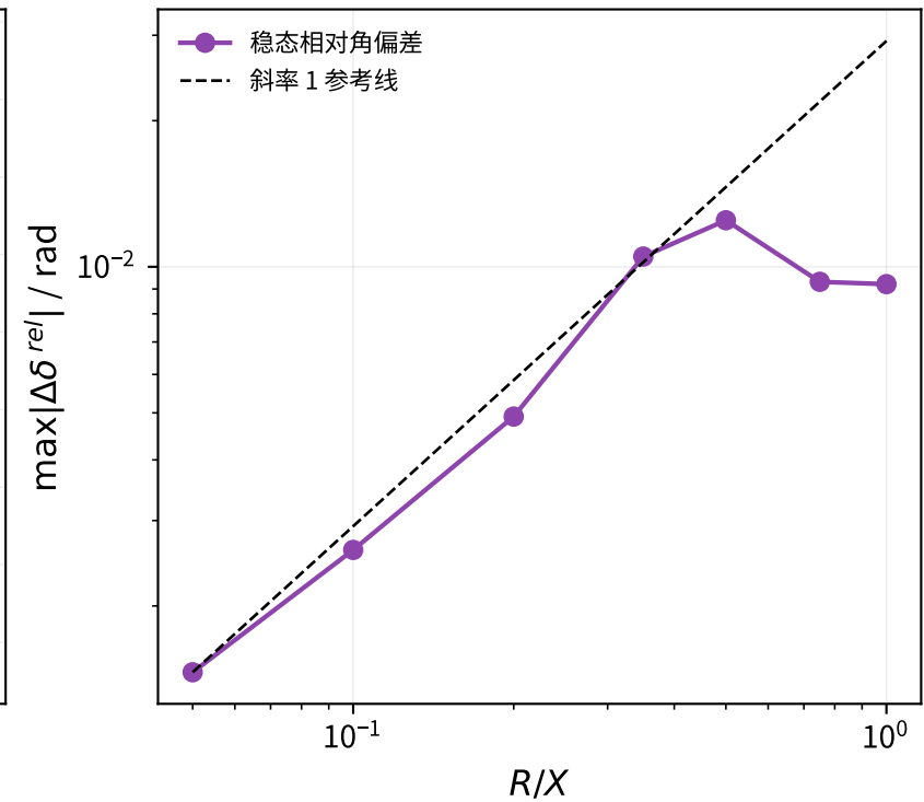
(c) 相对角偏差 \propto R/X : Kuramoto 丢掉的是电导 G 项
