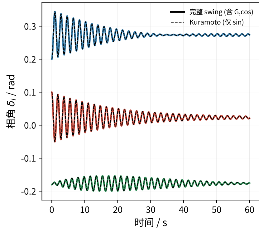
(a) R = 0 (无损纯感): 两者完全重合
