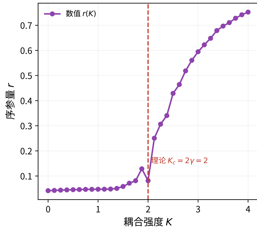
(a) 同步相变: r > 0 仅当 K > K_c
