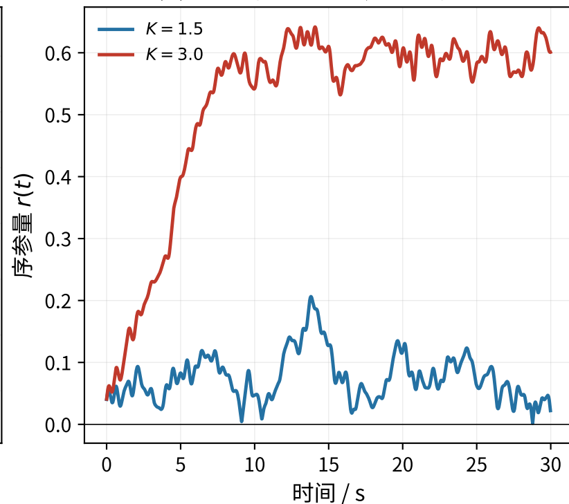
(b) K < K_c 趋向无序, K > K_c 同步
