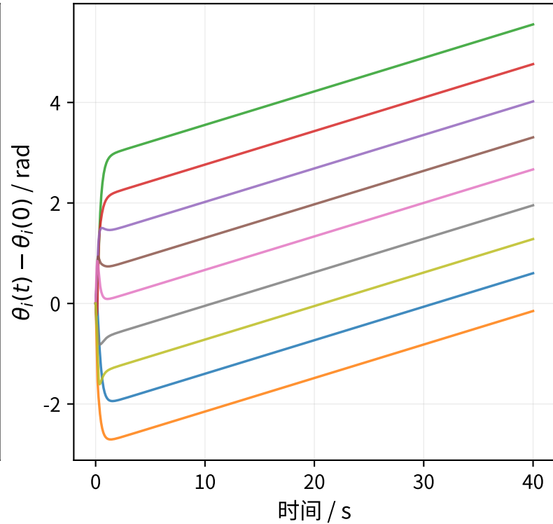
(c) K = 8 : 各节点相角锁定为同一斜率
