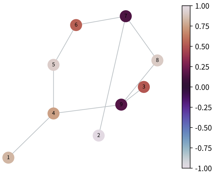
(a) IEEE 9 节点: 弱耦合 ( K = 0.5 ) 下相位分散
