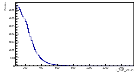
L_END_VRHO
