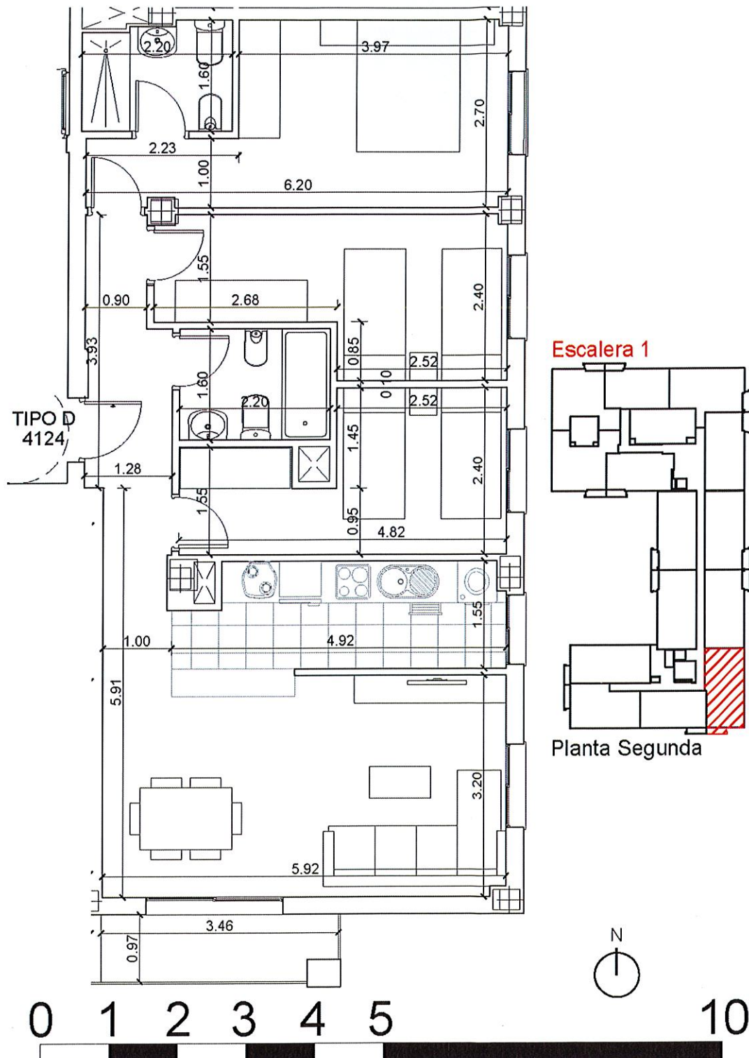
DISTRIBUCIÓN ESCALERA 1 Vivienda 4124. Tipo D
