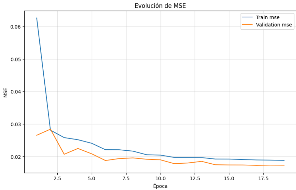
Figura 6.2: Gráfica de la evolución del MSE
