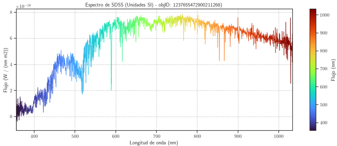
Figura 2.1: Ejemplo de espectro estelar observado por SDSS
