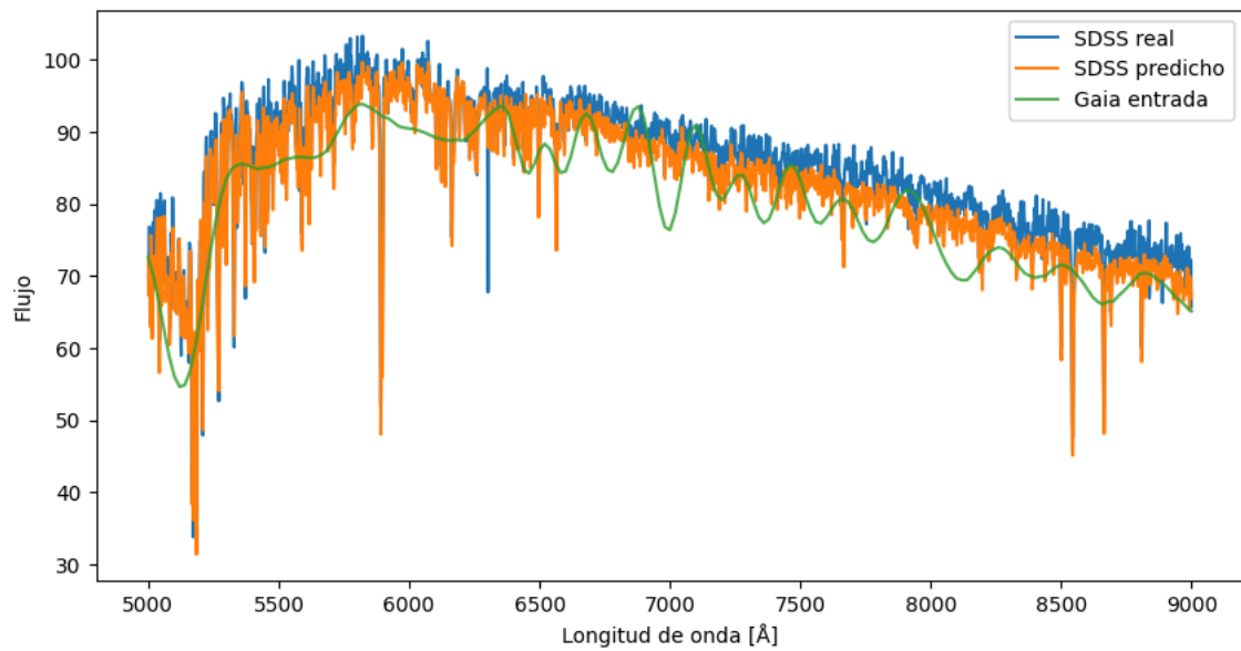
Figura 6.5: Ejemplo 2 del espectro generado por el modelo y los de Gaia y SDSS originales
