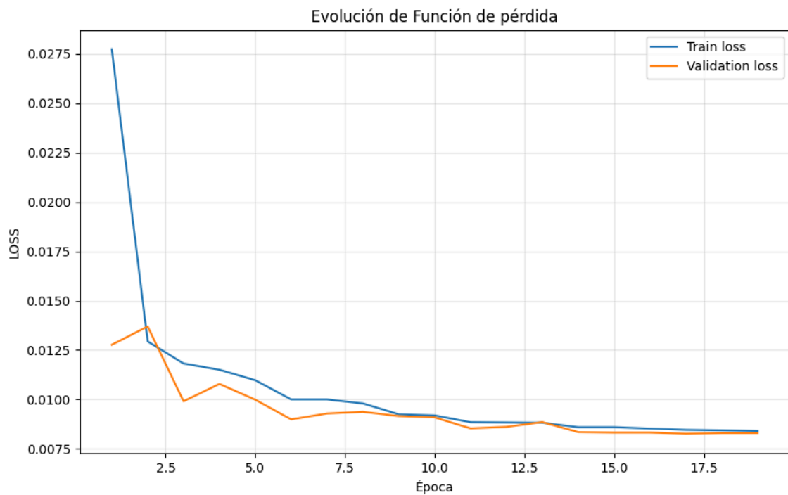
Figura 6.1: Gráfica de la evolución de la función de pérdida
