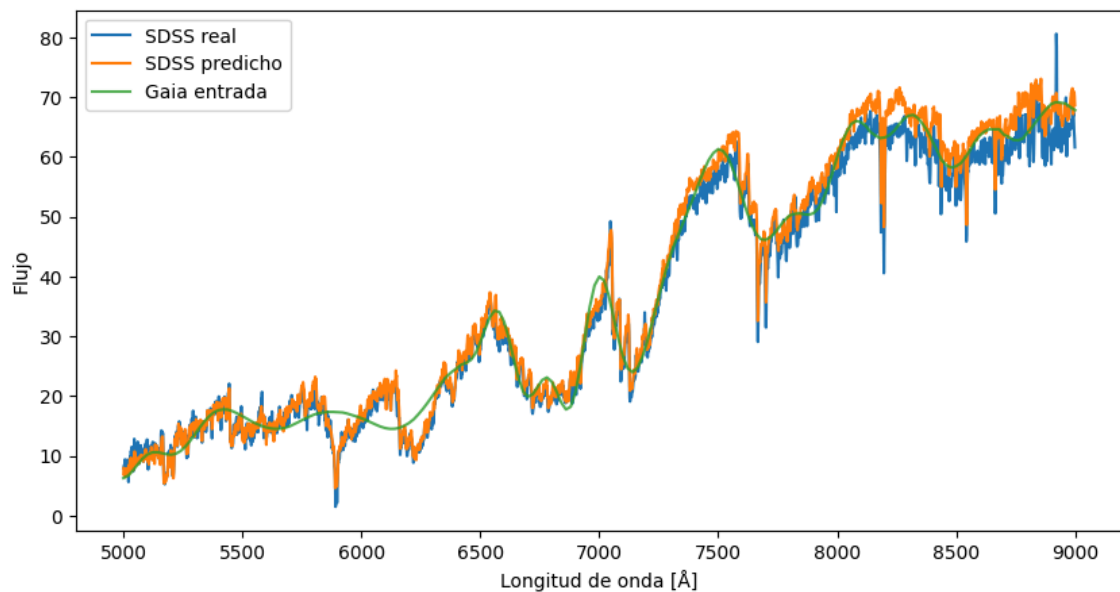
Figura 6.4: Ejemplo 1 del espectro generado por el modelo y los de Gaia y SDSS originales
