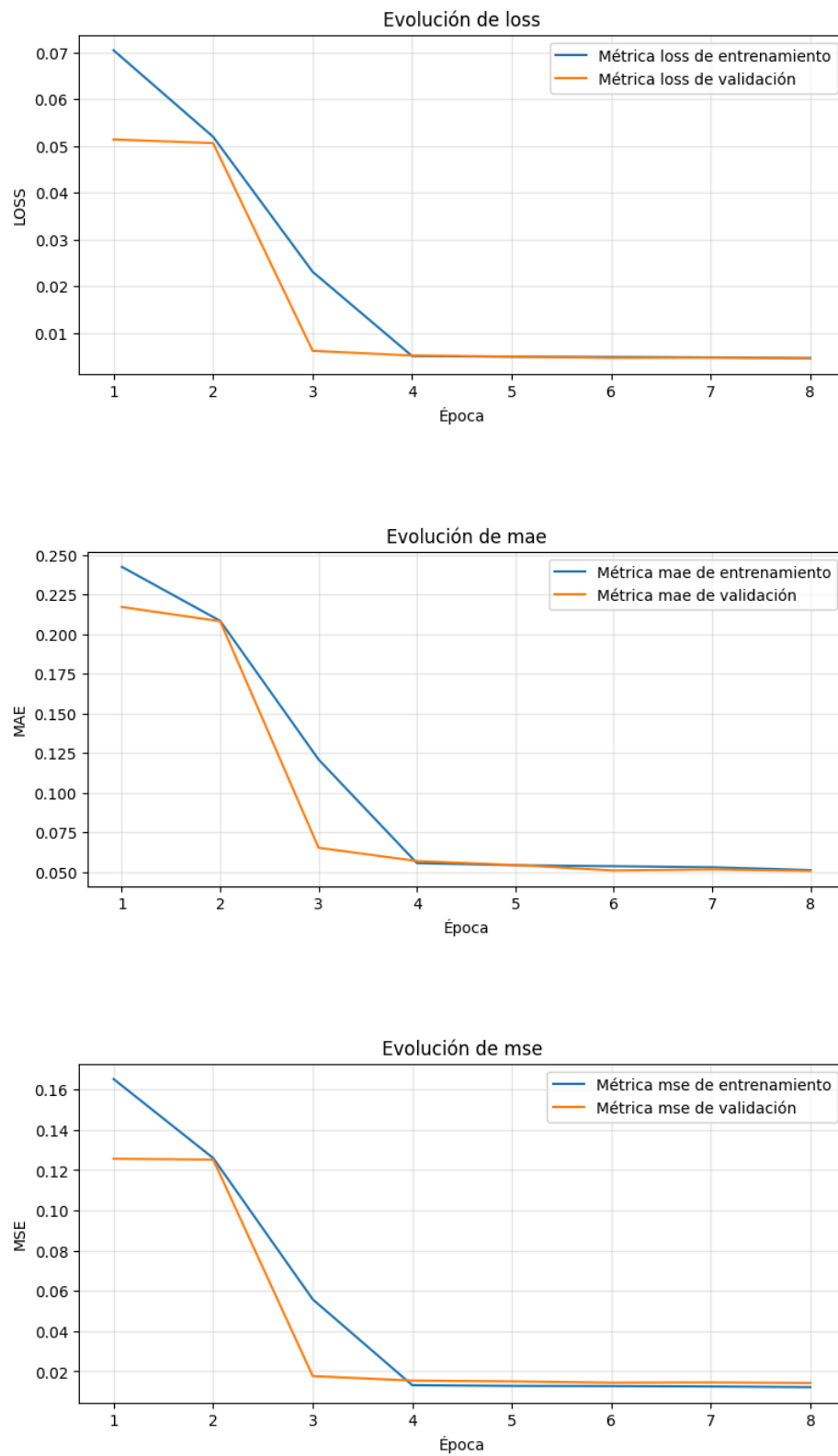
Figura 5.44. Gráficas de la evolución de las métricas de entrenamiento del modelo basado en el mecanismo de Atención
