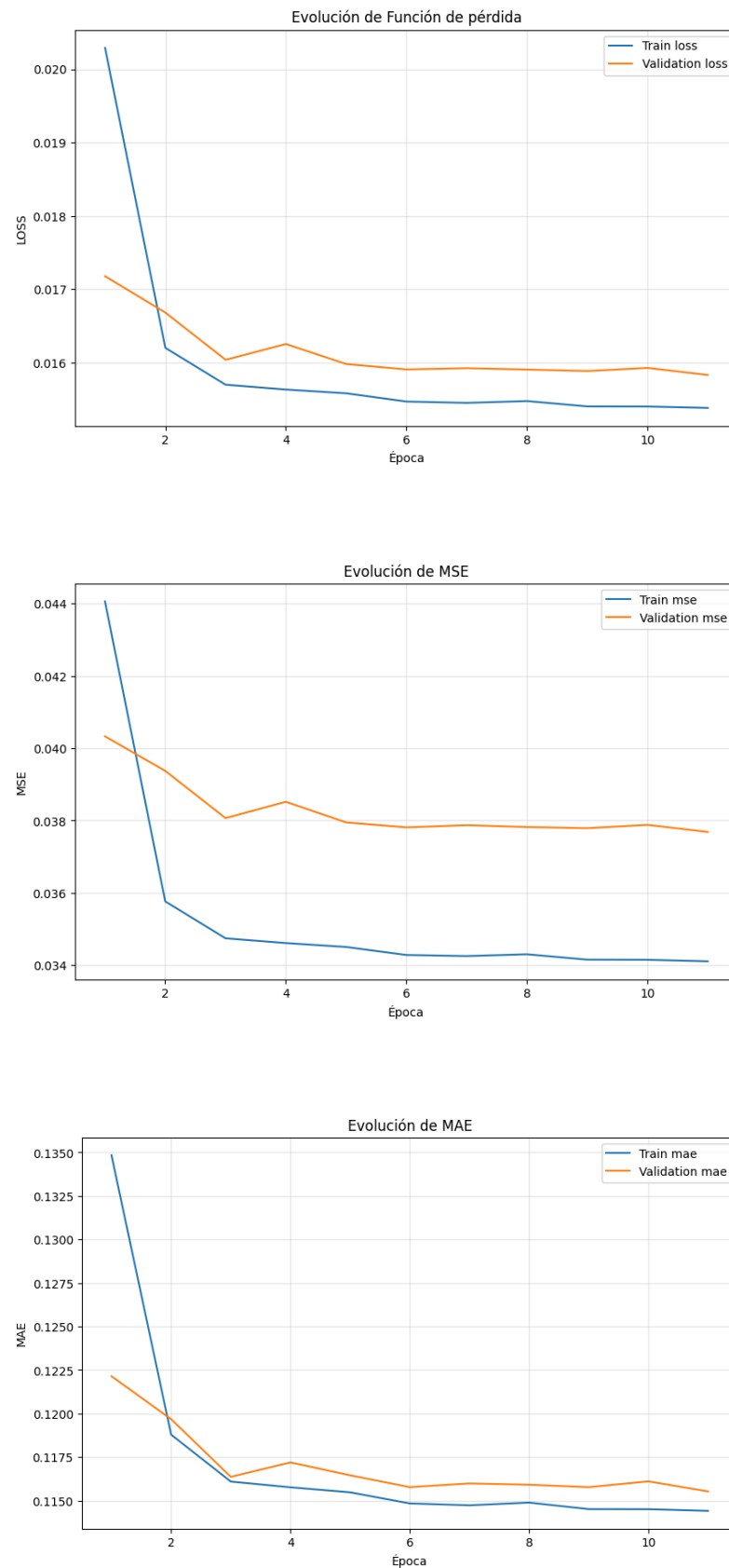
Figura 5.20. Gráficas de las métricas de evolución de entrenamiento en el modelo convolucional 1D
