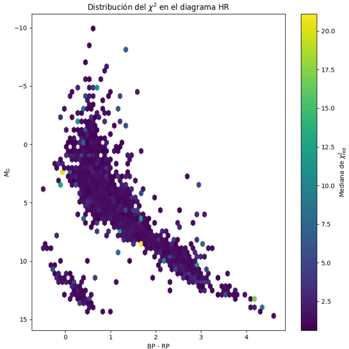
Figura 6.1. Diagrama HR del estadístico chi-cuadrado normalizado aplicado sobre la muestra de test en el modelo denso.
