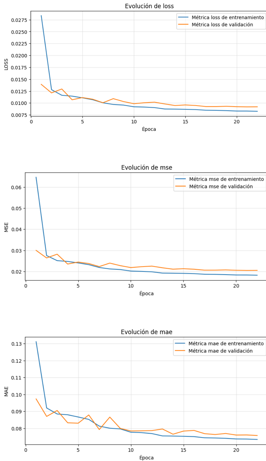
Figura 5.1. Gráfica de la evolución del MAE en el modelo de redes neuronales densas con normalización global.
