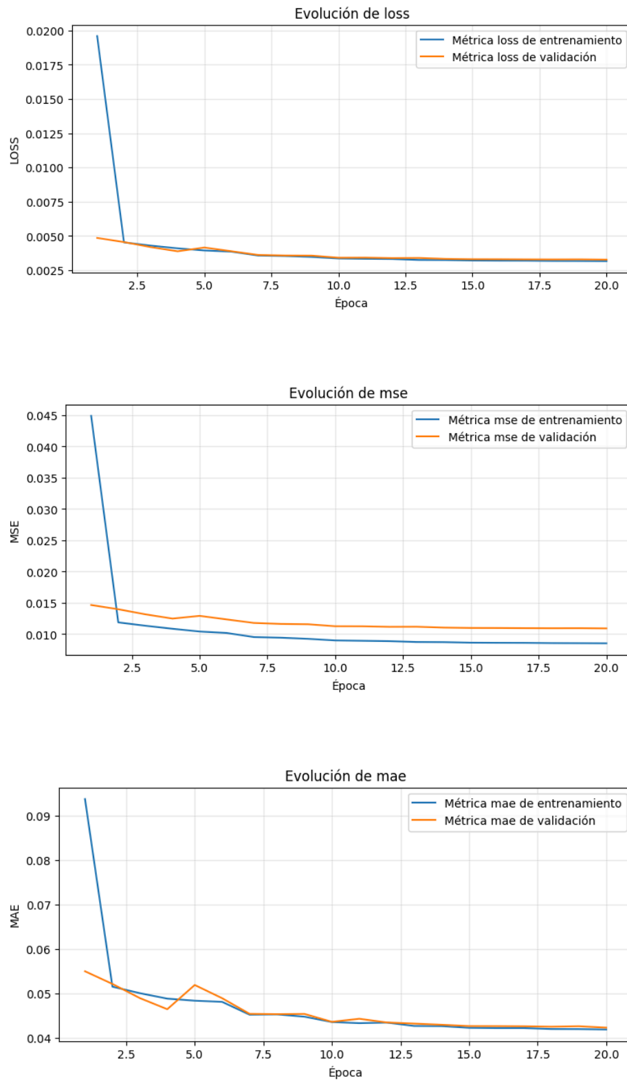
Figura 5.6. Gráficas de evolución de las métricas de entrenamiento en la red densa.
