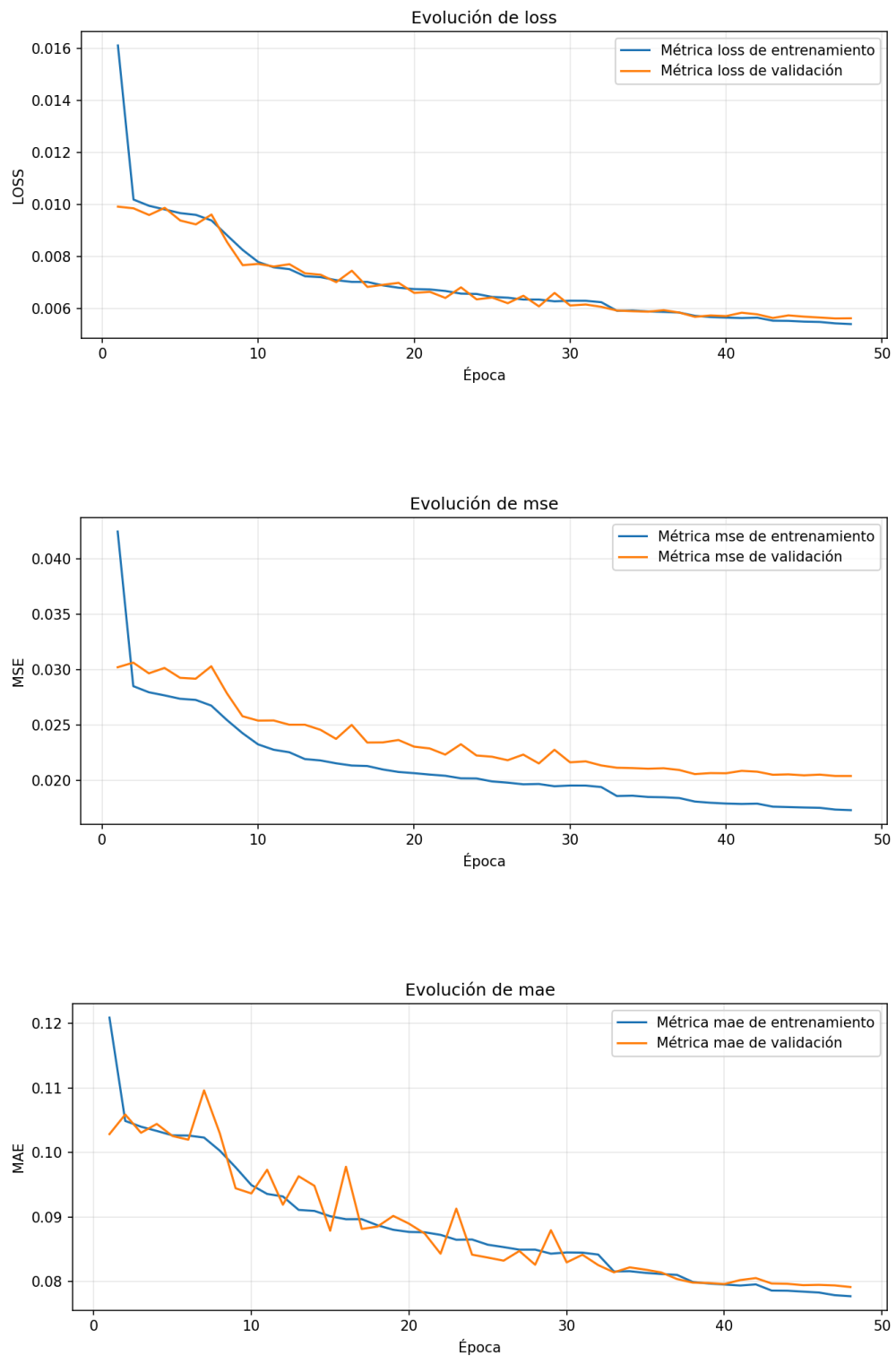
Figura 5.25. Gráficas de la evolución de las métricas de entrenamiento del modelo convolucional U-Net
