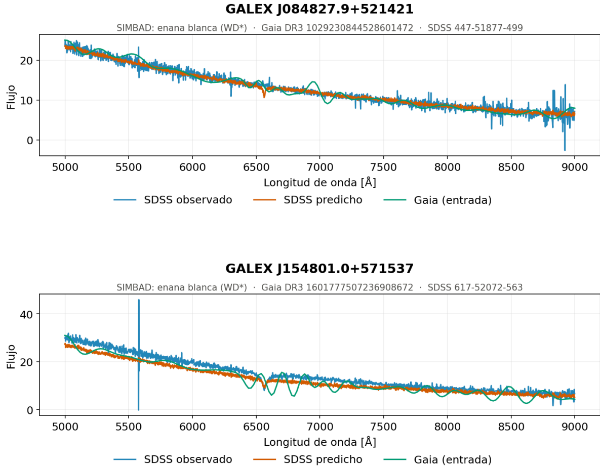
Figura 5.5. Enanas blancas. Espectros generados por el modelo de redes neuronales densas con normalización global para las enanas blancas, objetos calientes y poco luminosos cuyo espectro es un continuo decreciente con muy pocos rasgos.
