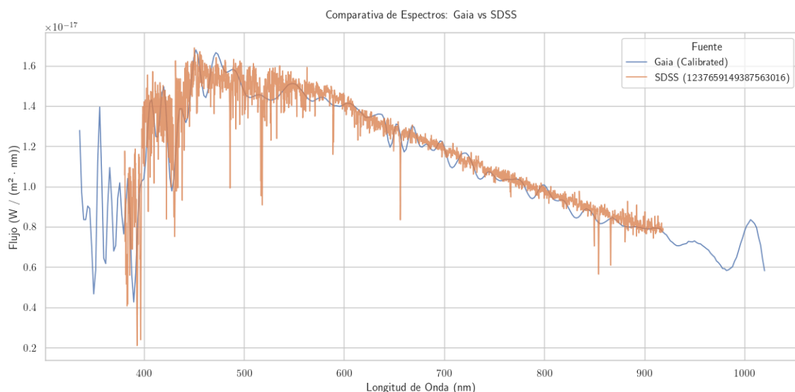
Figura 3.2: Ejemplo aleatorio del espectro captado de un mismo cuerpo por Gaia y SDSS
