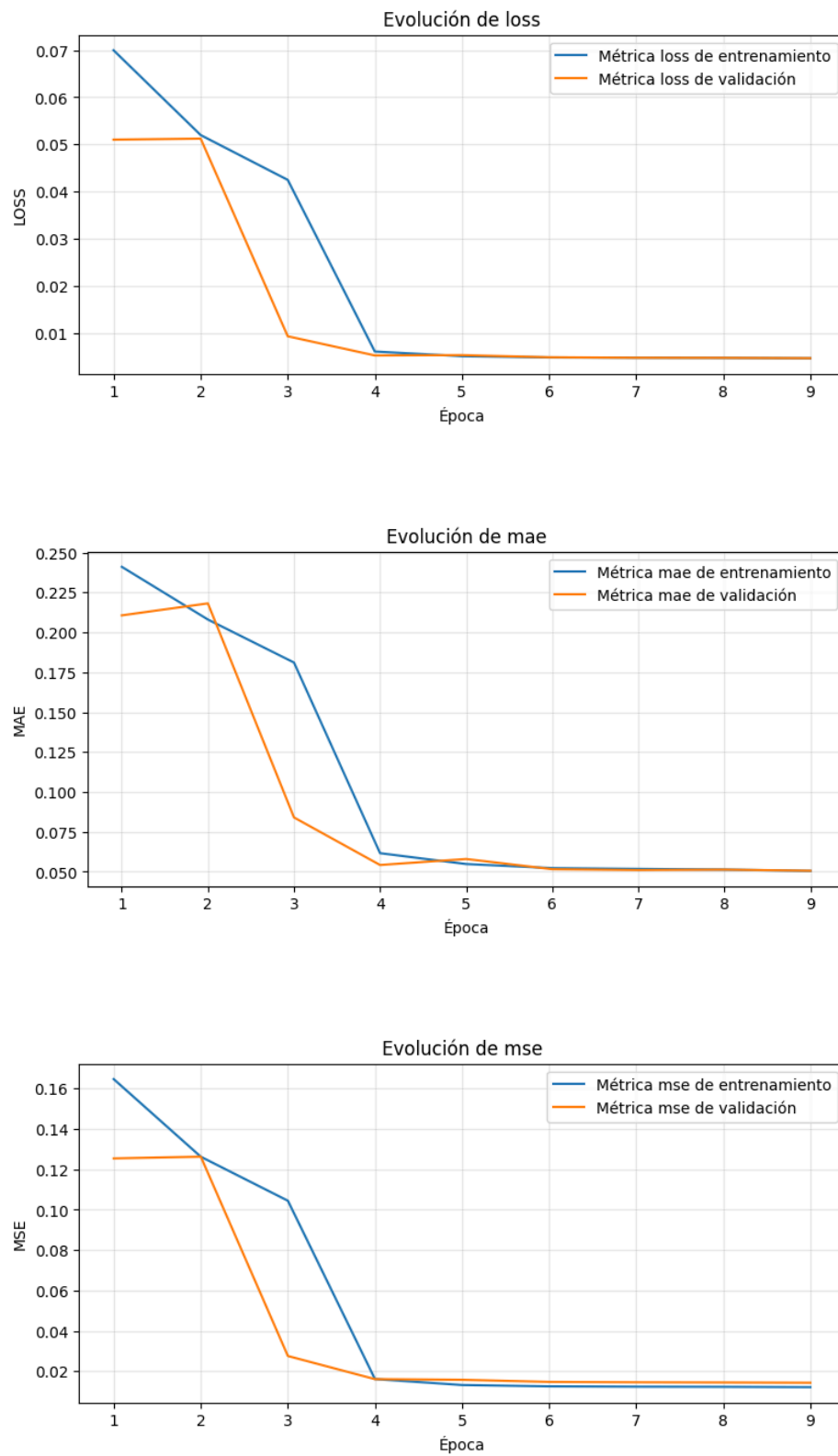
Figura 5.45. Gráficas de la evolución de las métricas de entrenamiento del modelo basado en el mecanismo de Atención
