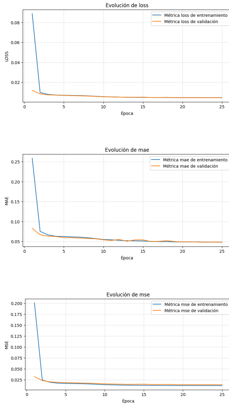
Figura 5.35. Gráficas de la evolución de las métricas de entrenamiento del modelo basado en una capa GRU
