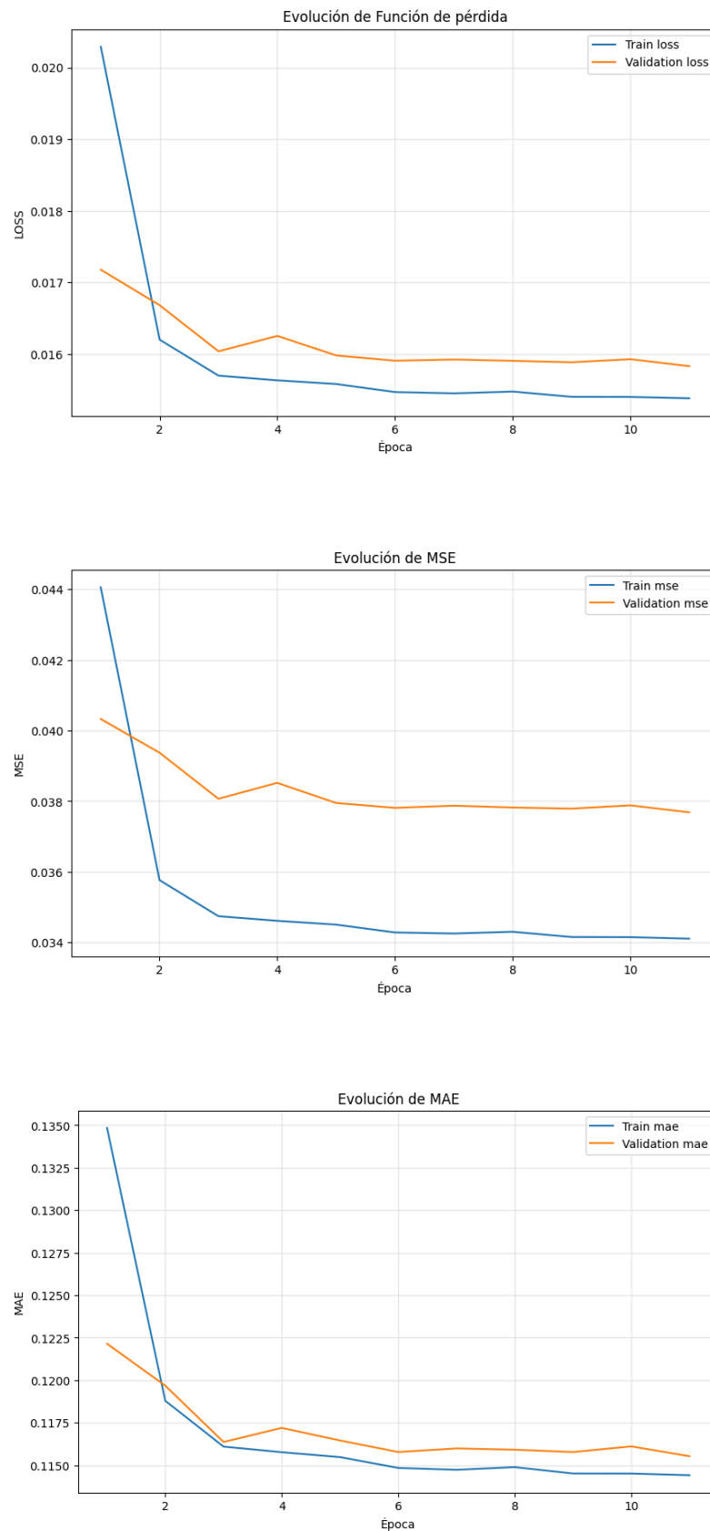
Figura 5.21. Gráficas de las métricas de evolución de entrenamiento en el modelo convolucional 1D
