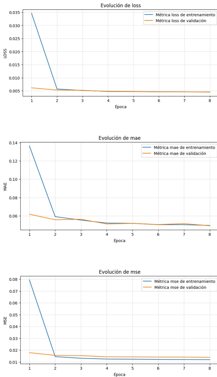
Figura 5.40. Gráficas de la evolución de las métricas de entrenamiento del modelo basado en una capa Bidireccional
