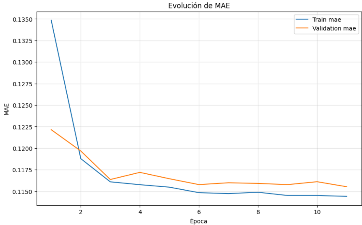
Figura 6.20. Gráfica de la evolución del MAE del modelo convolucional 1D
