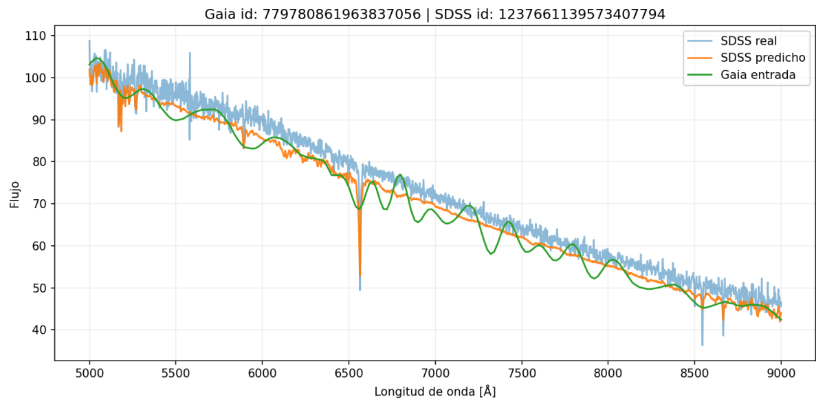
Figura 6.27. Ejemplo 2 del espectro generado por el modelo convolucional U-Net.
