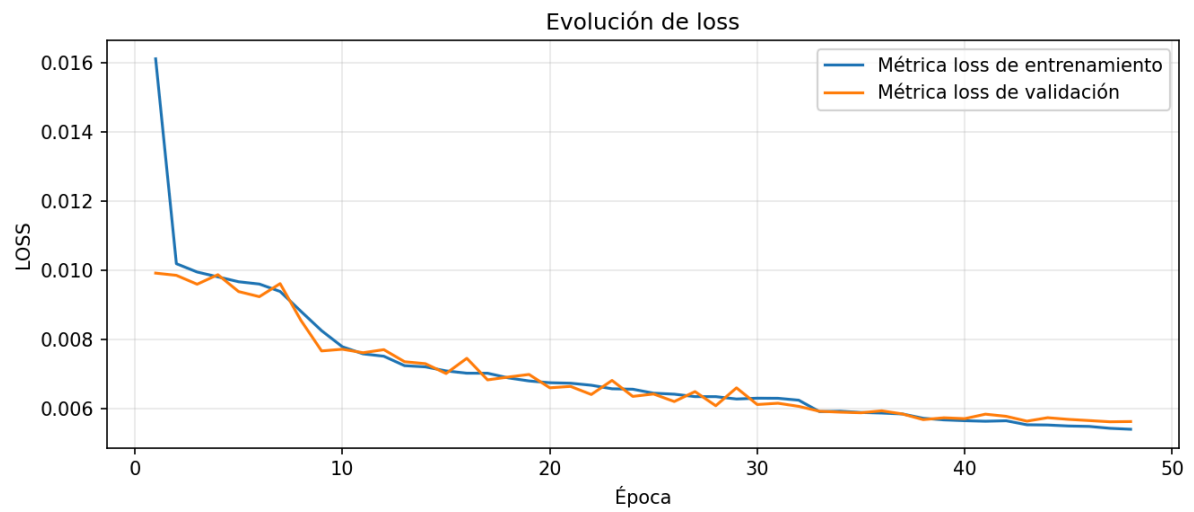
Figura 6.23. Gráfica de la evolución de la función de pérdida del modelo convolucional U-Net
