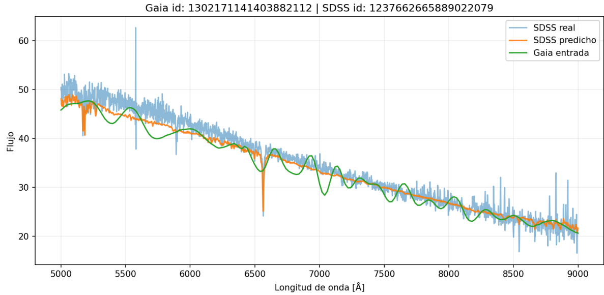
Figura 6.26. Ejemplo 1 del espectro generado por el modelo convolucional U-Net.
