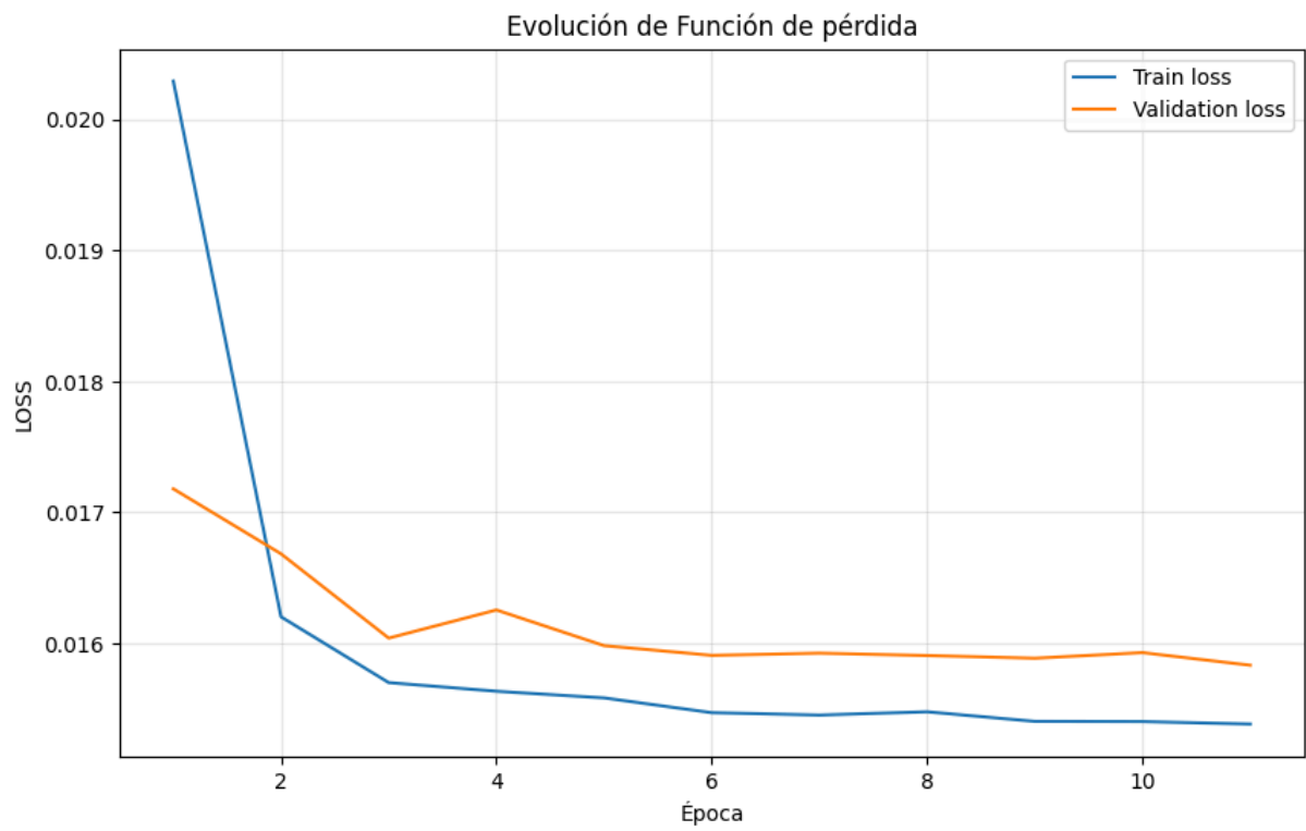
Figura 6.18. Gráfica de la evolución de la función de pérdida del modelo convolucional 1D
