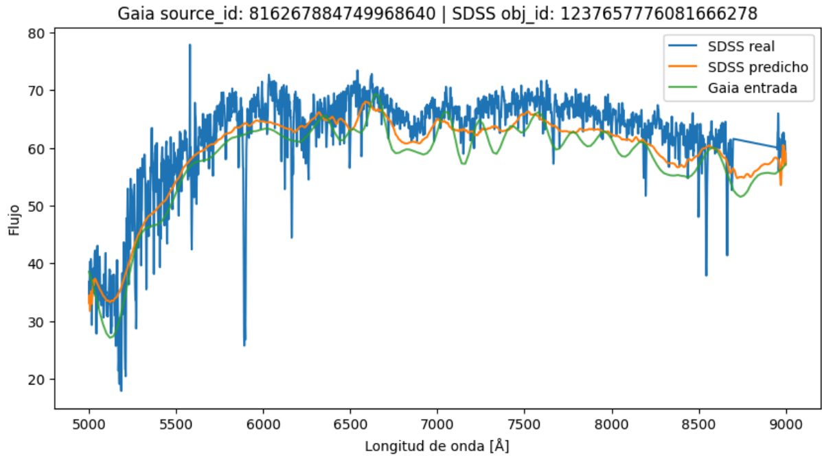
Figura 6.22. Ejemplo 2 del espectro generado por el modelo convolucional 1D.
