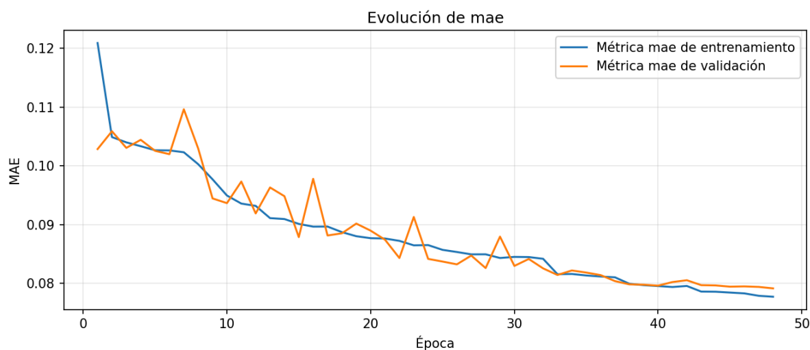
Figura 6.25. Gráfica de la evolución del MAE del modelo convolucional U-Net
