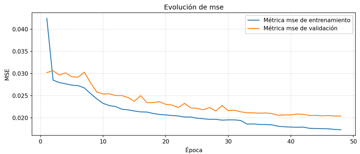
Figura 6.24. Gráfica de la evolución del MSE del modelo convolucional U-Net
