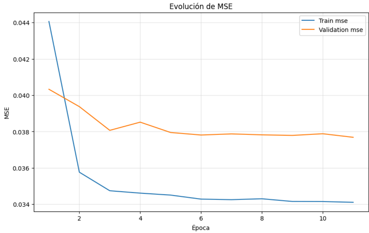
Figura 6.19. Gráfica de la evolución del MSE del modelo convolucional 1D
