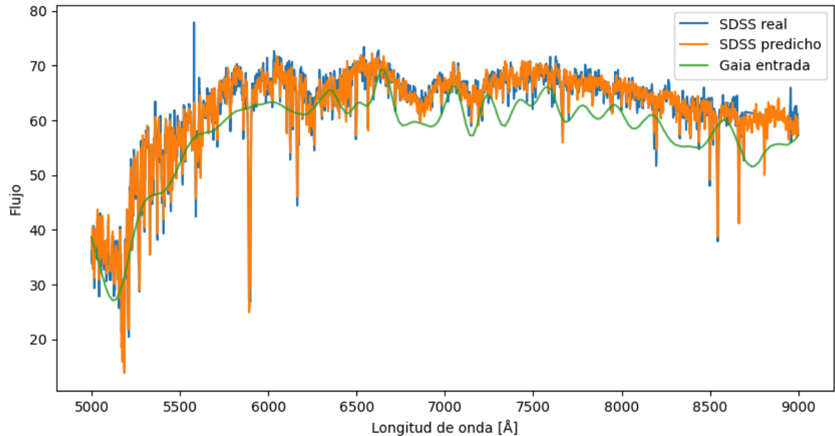
Figura 6.17. Ejemplo 2 del espectro generado por el modelo de redes neuronales densas con la variable SNR como entrada.
