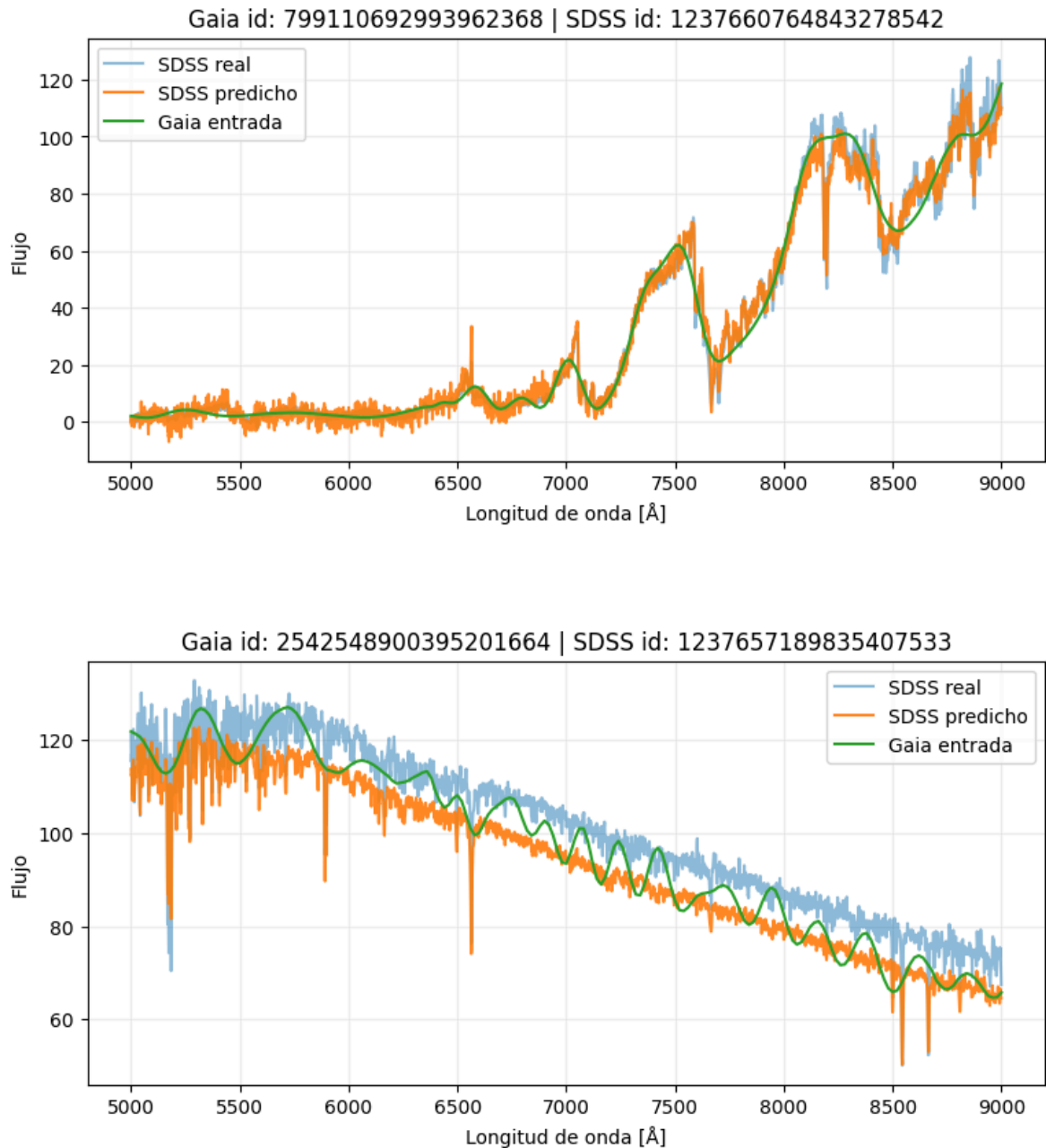
Figura 6.5. Ejemplos de espectros generados por el modelo de redes neuronales densas con normalización basada en el máximo de cada espectro.
