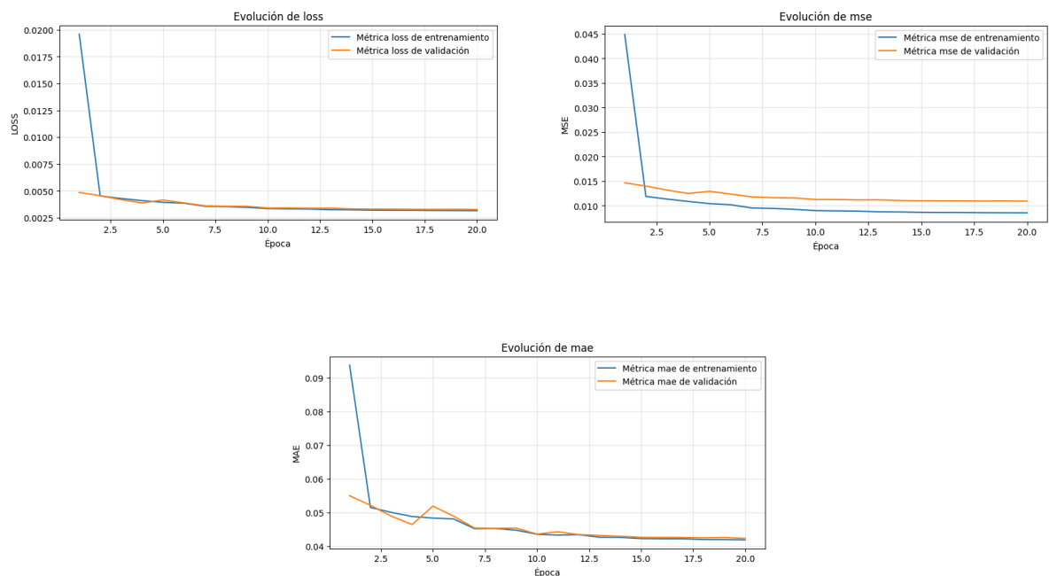
Figura 6.3. Gráficas de evolución de las métricas de entrenamiento en la red densa.
