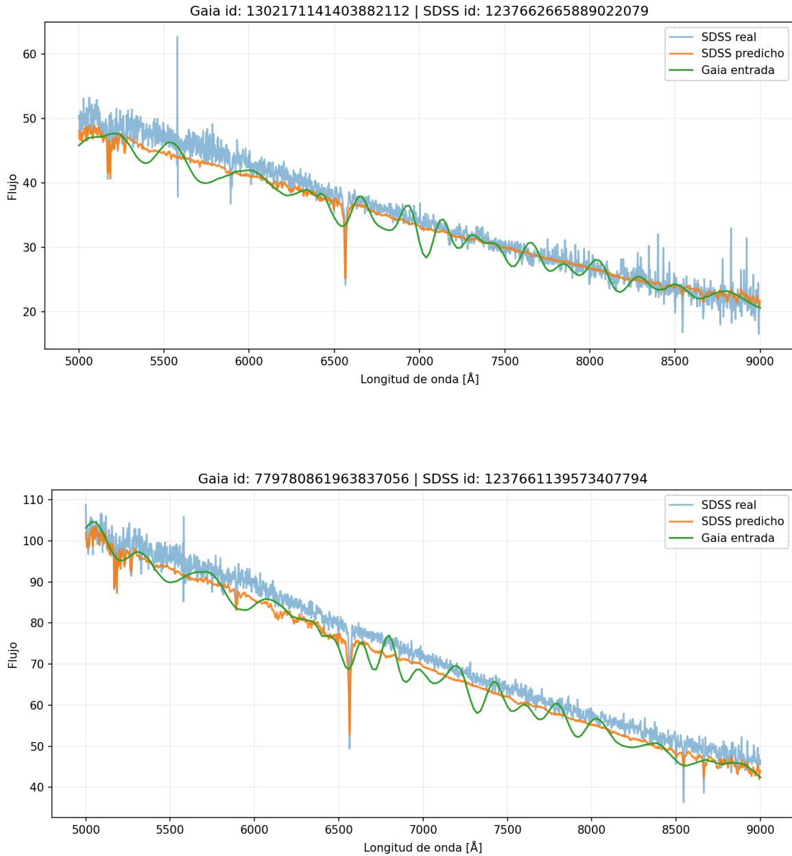
Figura 6.11. Ejemplos de espectros generados por el modelo convolucional U-Net.
