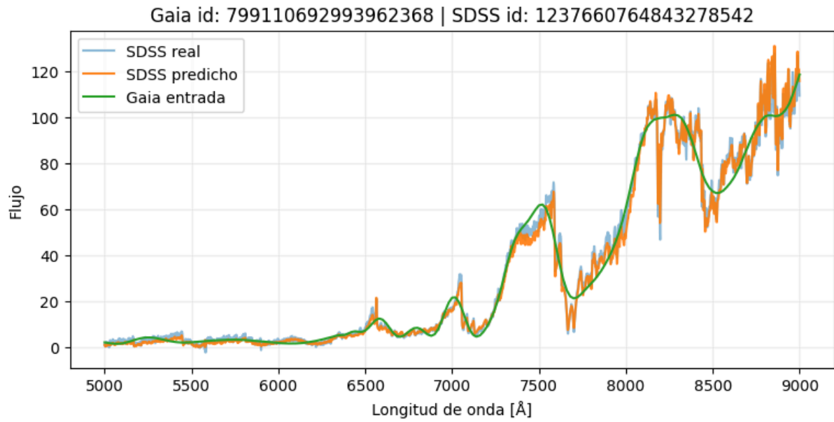
Figura 6.12. Ejemplo 1 del espectro generado por el modelo de redes neuronales recurrentes con una capa de GRU.
