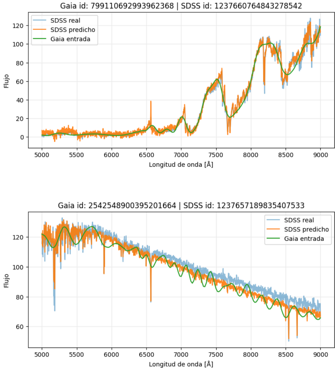
Figura 6.2. Ejemplos de espectros generados por el modelo de redes neuronales densas con normalización basada en la mediana del conjunto de entrenamiento.
