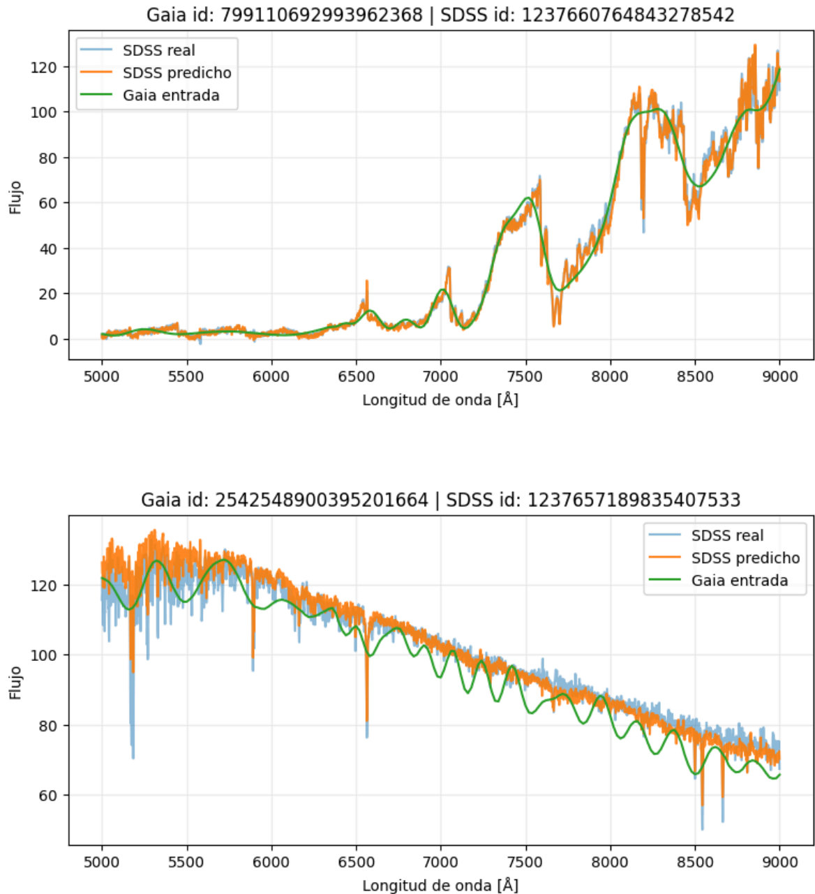
Figura 6.7. Ejemplos de espectros generados por el modelo de redes neuronales densas con la variable SNR como entrada.
