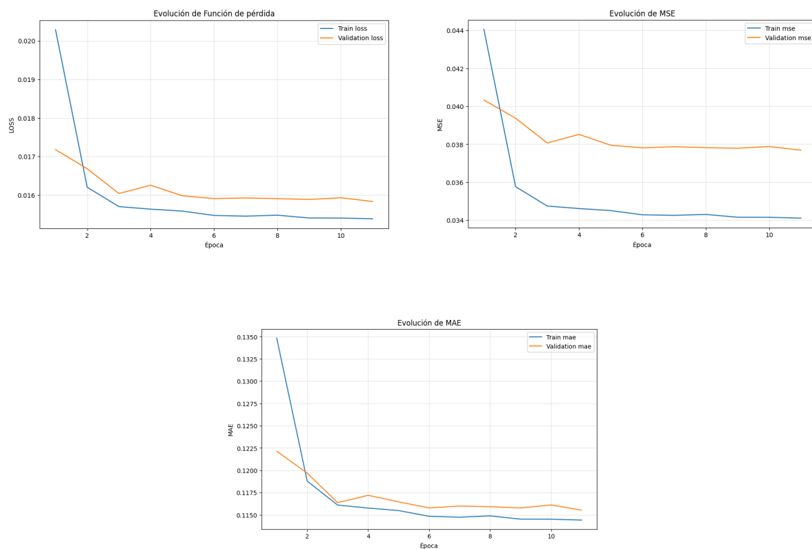
Figura 6.8. Gráficas de las métricas de evolución de entranamiento en modelo convolucional 1D
