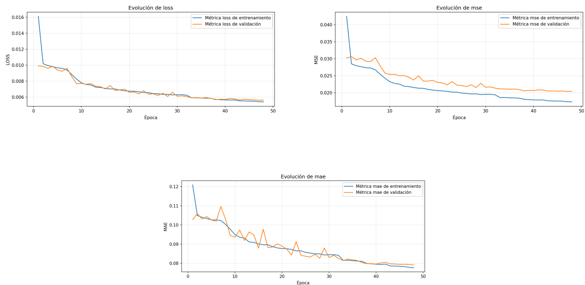
Figura 6.10. Gráficas de la evolución de las métricas de entrenamiento del modelo convolucional U-Net
