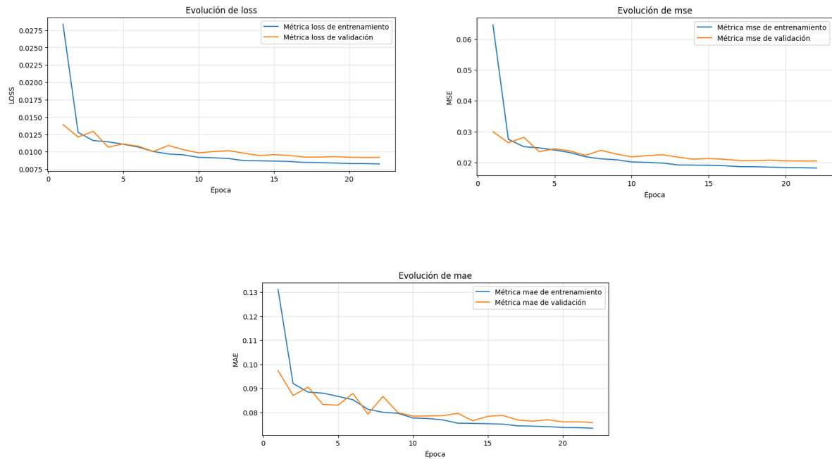
Figura 6.1. Gráfica de la evolución del MAE en el modelo de redes neuronales densas con normalización global.
