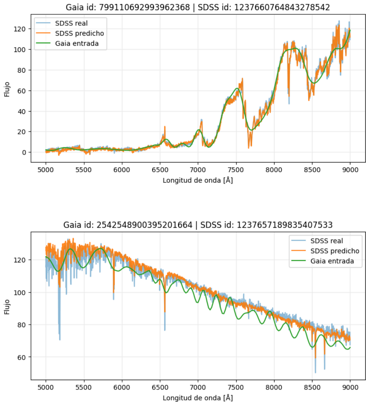
Figura 6.15. Ejemplos de espectros generados por el modelo de redes neuronales recurrentes con una función de Atención.
