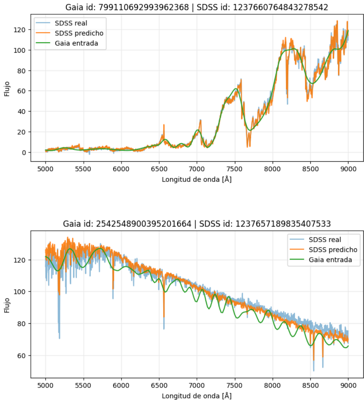
Figura 6.4. Ejemplos de espectros generados por el modelo de redes neuronales densas con normalización basada en la mediana de cada espectro.
