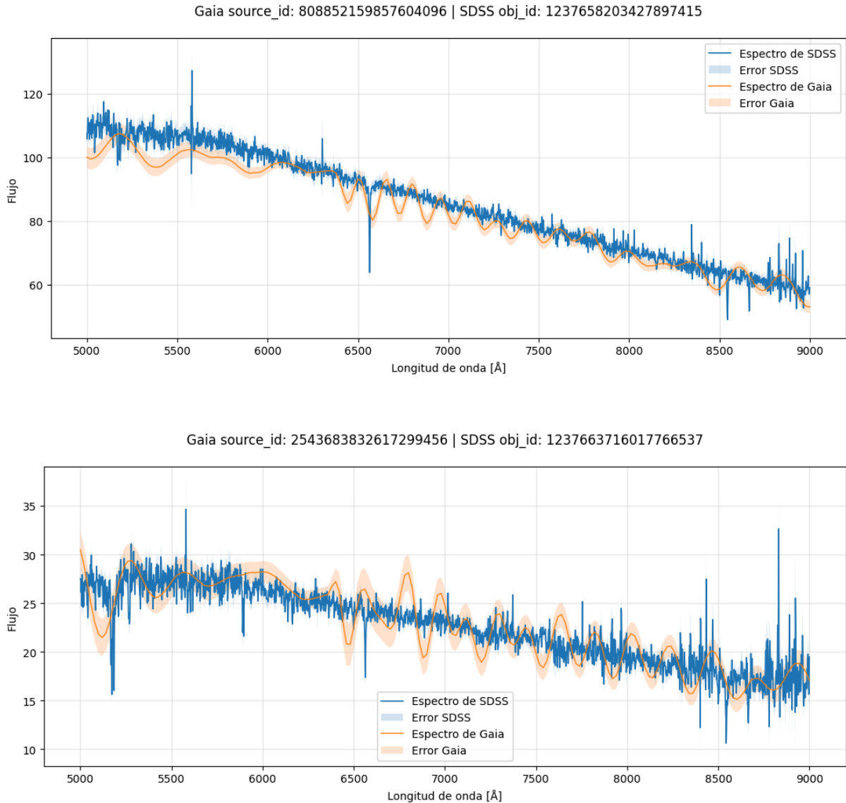
Figura 5.5. Ejemplos de los espectros observados por Gaia y SDSS con bandas de error
