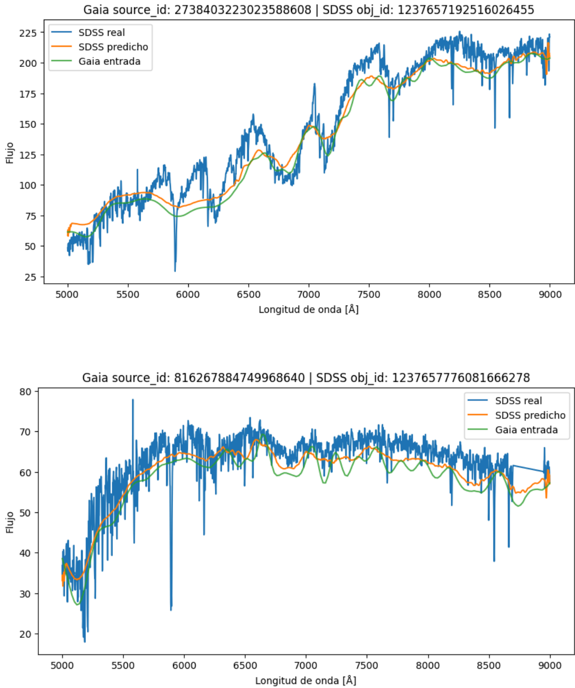
Figura 6.9. Ejemplos de espectros generados por el modelo convolucional 1D.
