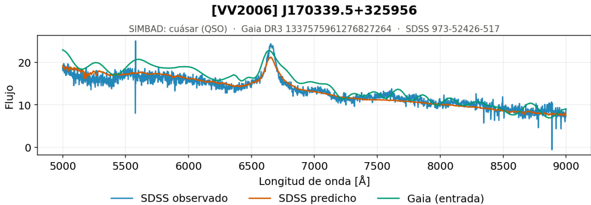
Figura 5.59. Secuencia central, alta luminosidad y alta temperatura, ejemplo 2. Espectro generado por el modelo convolucional U-Net para uno de los objetos con paralaje no significativo, por debajo de 0,01 mas, cuya magnitud absoluta no es fiable: SIMBAD lo identifica como un QSO, y no como una estrella de la secuencia principal.
