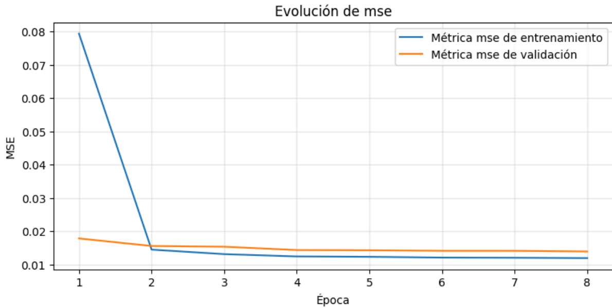
Figura 5.87. Evolución del MSE durante el entrenamiento del modelo basado en una capa Bidireccional
