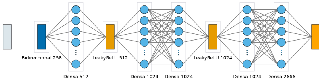
Figura 4.13. Arquitectura del modelo recurrente bidireccional
